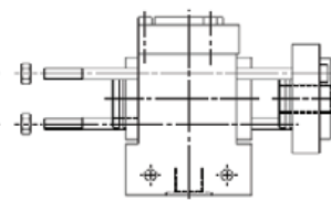
модуль с заглушкой
