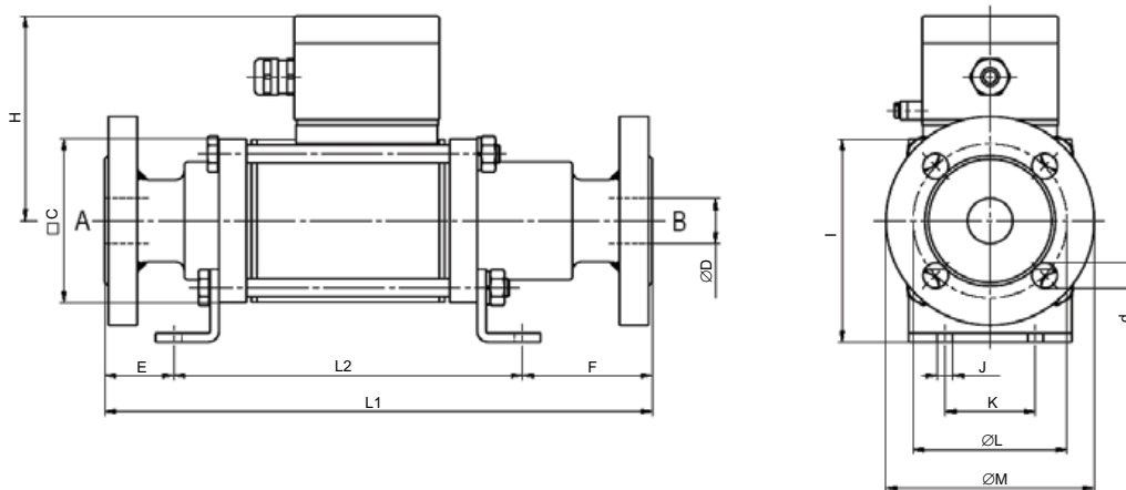
ГАБАРИТНЫЕ РАЗМЕРЫ, (мм)
