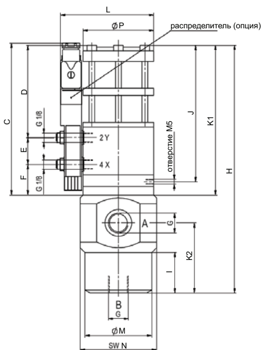
Серия PCS-3 с картриджем
