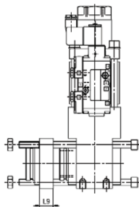
удлинненный модуль с разделительной плитой
