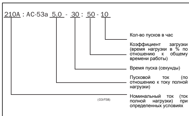
Рис. 8 Описание типоразмера по норме АС53а
