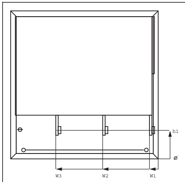
Рис. 21 Размеры шин MSF-310 ... MSF-835
