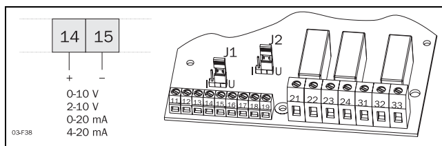
Рис. 37 Подключение аналогового сигнала
