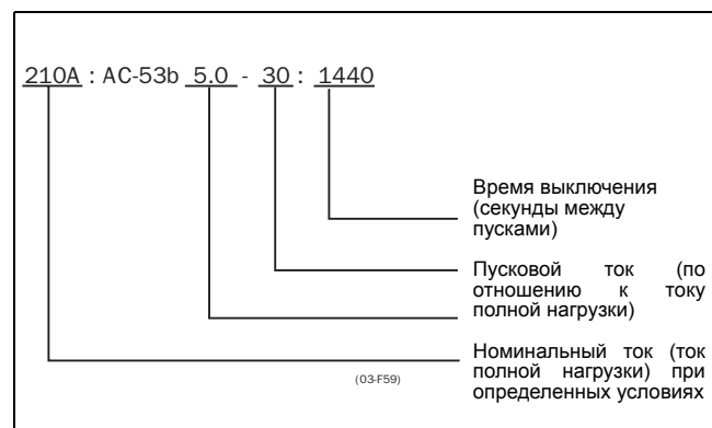
Рис. 10 Описание типоразмера по норме АС53b
