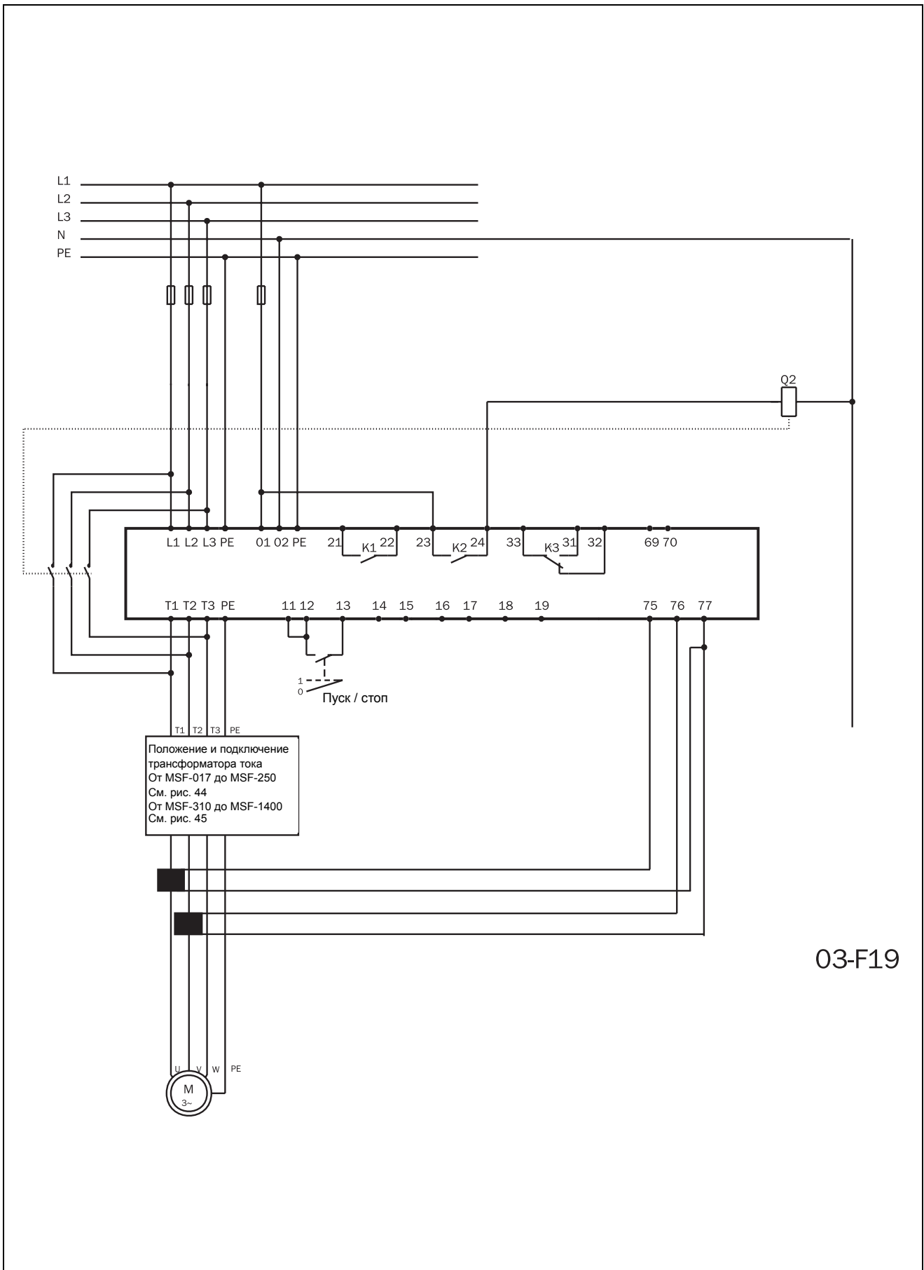
Рис. 43 Подключение с шунтированием для MSF 310-1400
