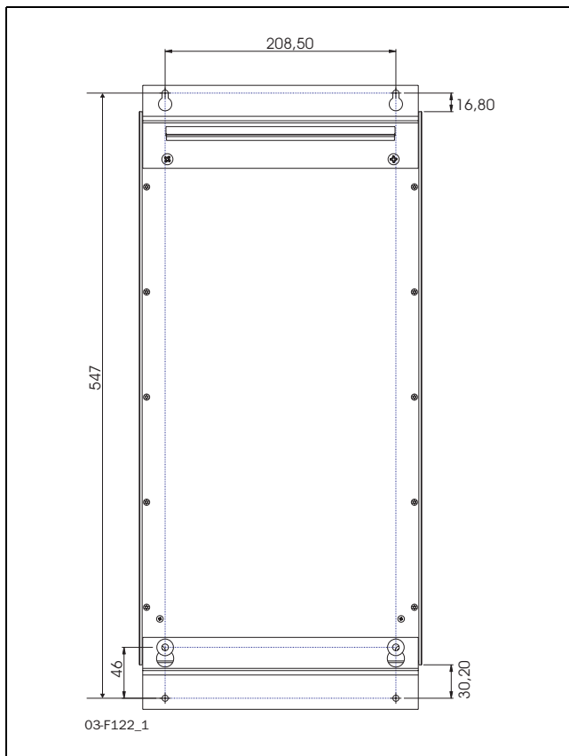
Рис. 18 Монтажные отверстия для MSF-170 ... MSF-250 с кронштейном верхнего крепления вместо DIN-направляющих.
