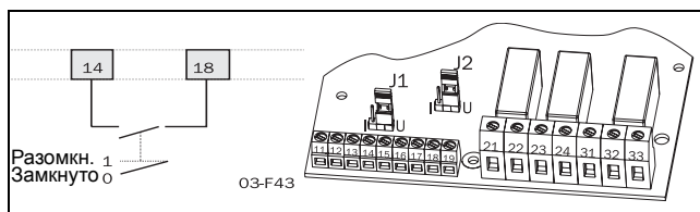
Рис. 54 Подключение внешнего сигнала управления медленной скоростью.
