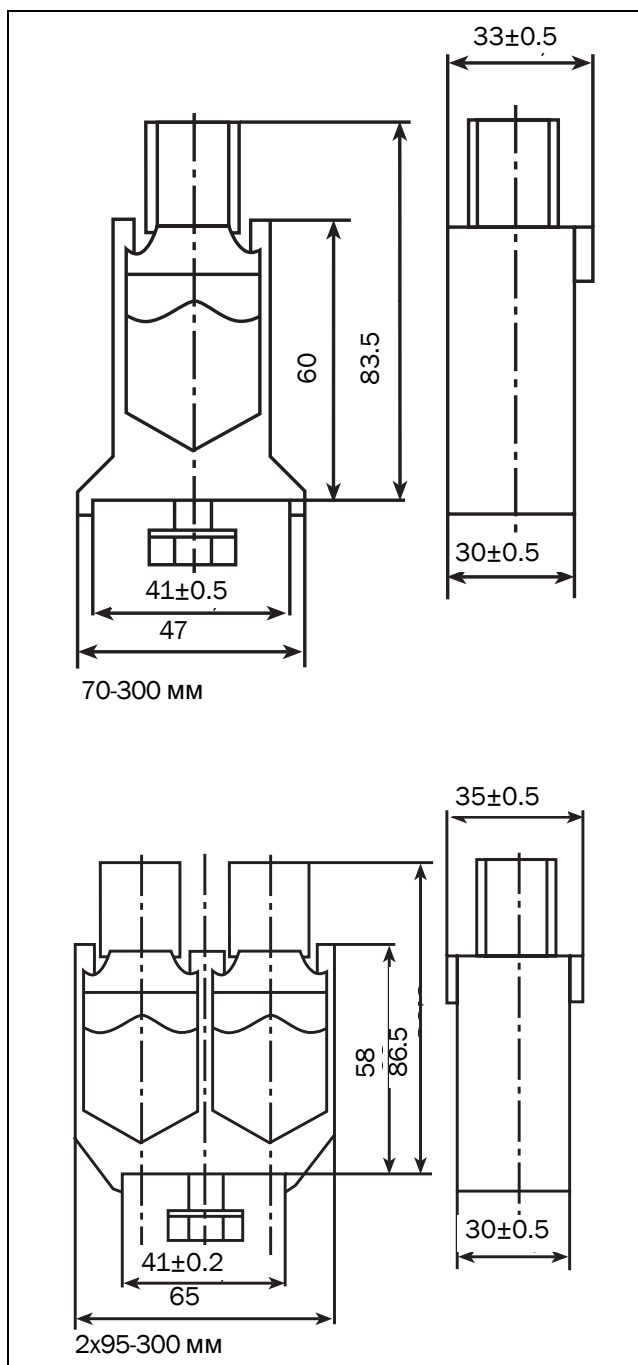
Рис. 64 Присоединительные клеммы
