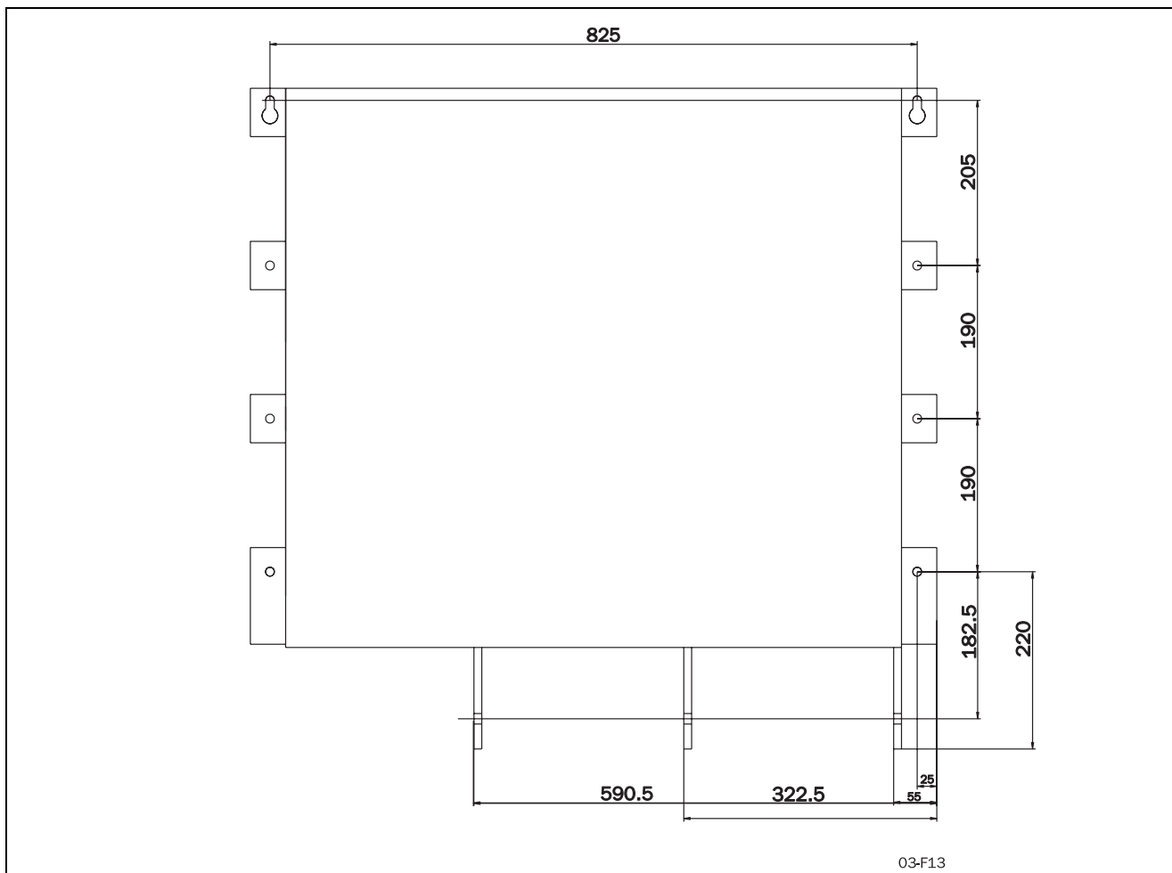
Рис. 23 Размеры отверстий для шин MSF-1000 ... MSF-1400
