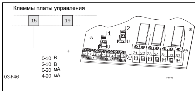
Рис. 51 Подключение аналогового выхода
