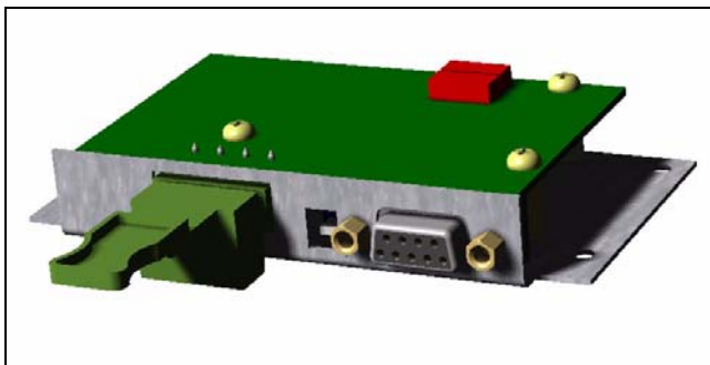
Рис. 60 60 Опция RS232 / RS485
