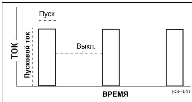
Рис. 11 Цикл работы, с шунтированием
