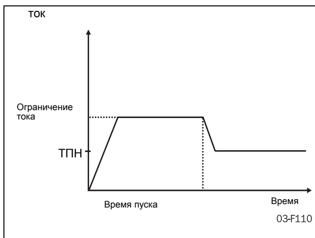
Рис. 35 Ограничение тока
