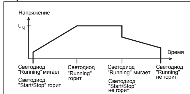
Рис. 14 Состояние светодиодов в различных режимах.
