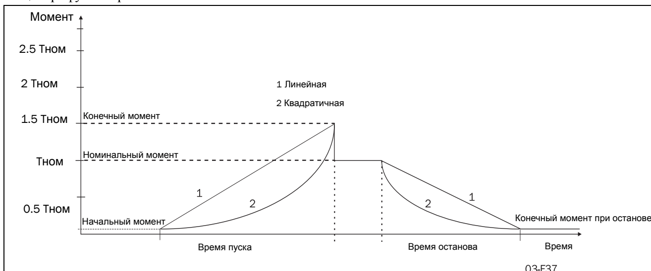
Рис. 40 Управление моментом при пуске и останове
