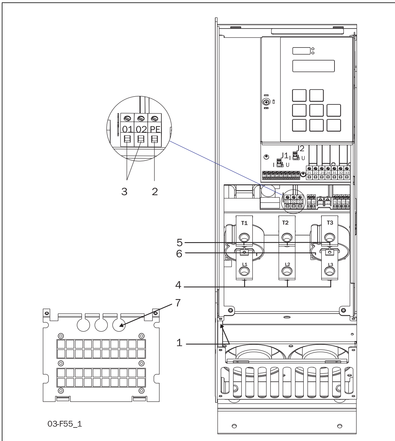
Рис. 25 Подключение MSF-110 ... MSF-145
