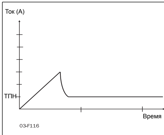
Рис. 7 График пуска при выборе управления напряжением
