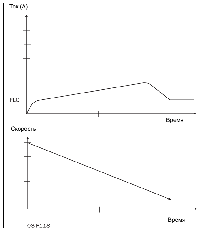
Рис. 36 Управление насосом
