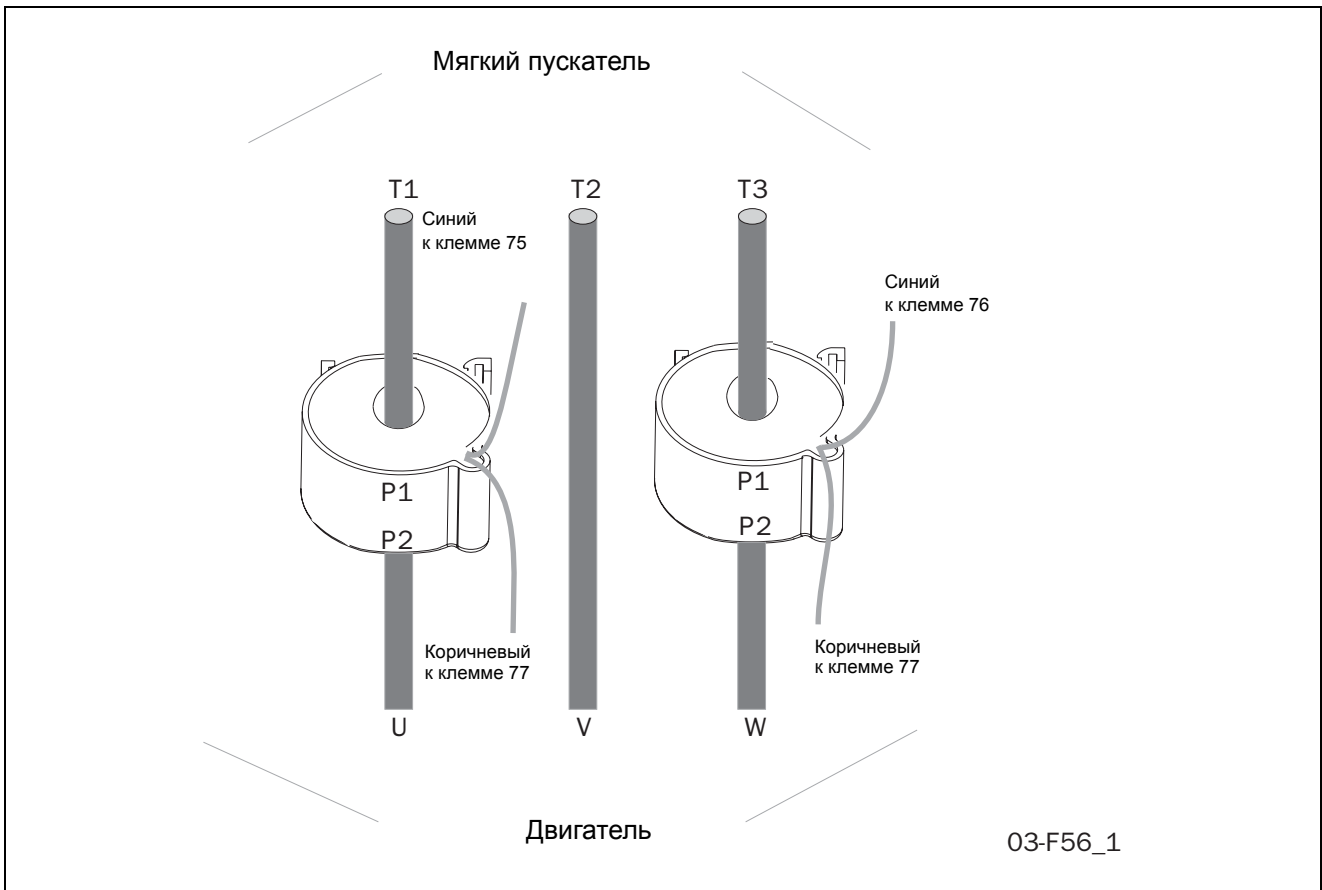
Рис. 44 Установка трансформаторов тока при шунтировании для MSF-017 ... MSF-250.
