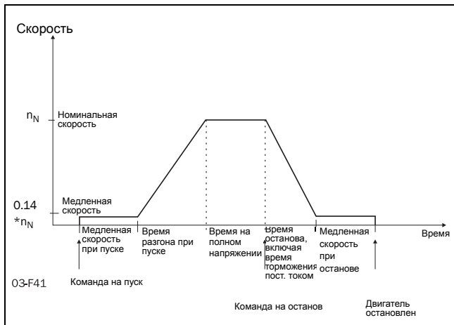
Рис. 49 Малая скорость при пуске/останове в течение выбранного времени
