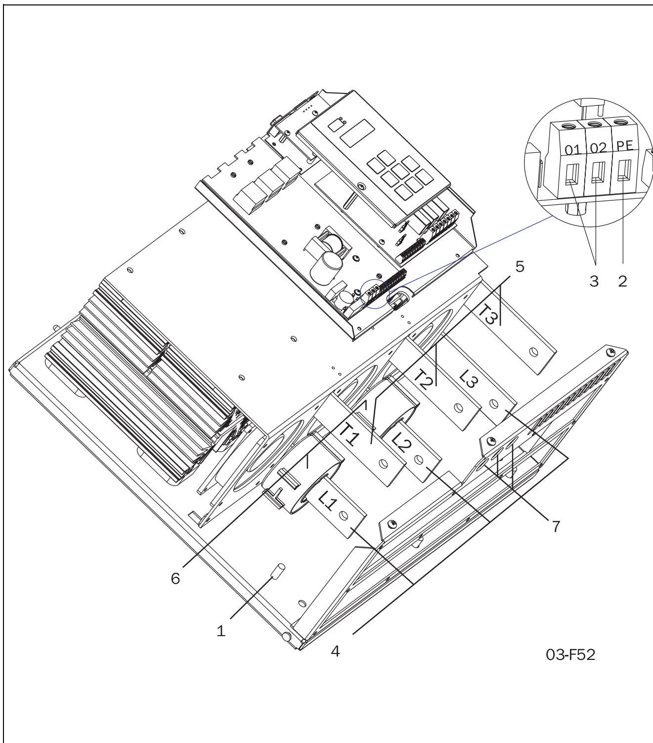
Рис. 27 Подключение MSF-310 ... MSF-1400
