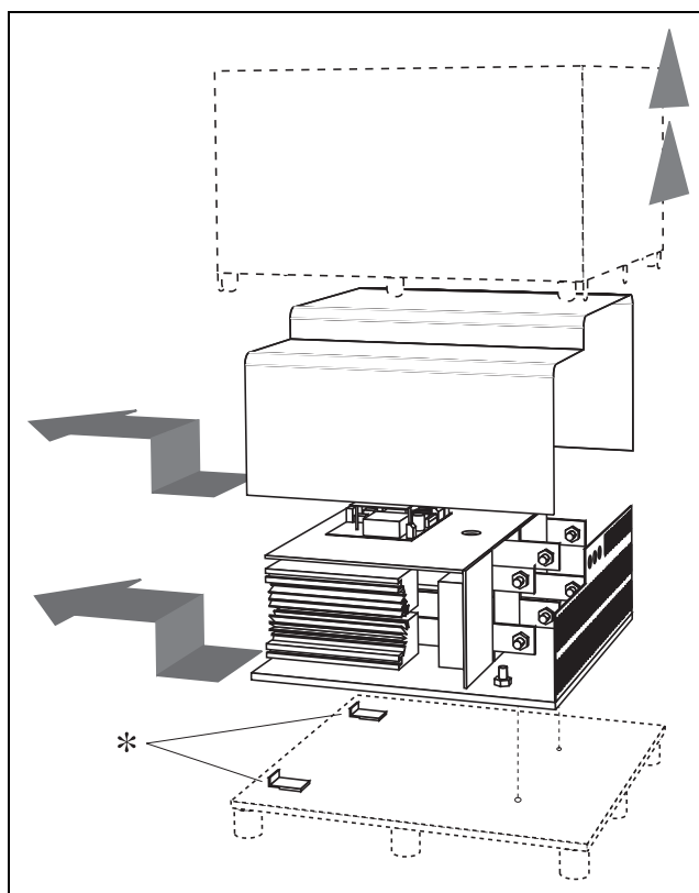
Рис. 2 Распаковка MSF-310 и больших типов
