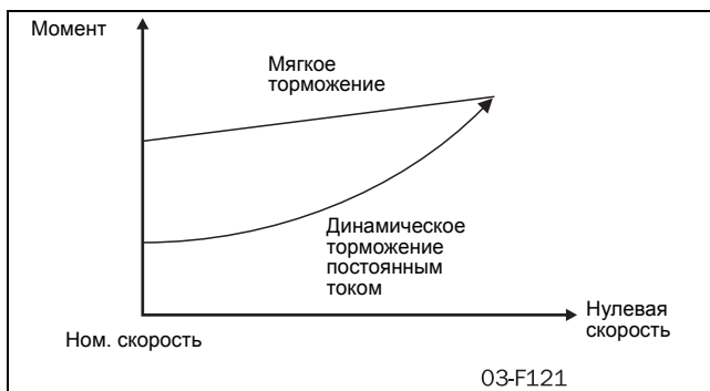
Рис. 46 Время торможения
