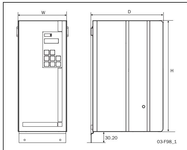
Рис. 16 Размеры MSF-017 ... MSF-250
