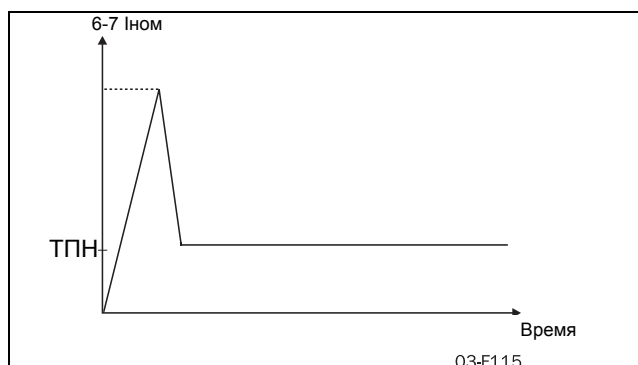
Рис. 39 Прямой пуск
