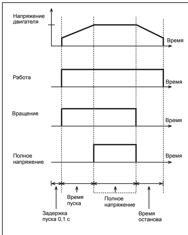
Рис. 50 Пуск/останов и функции реле "Работа" и "Полное напряжение"
