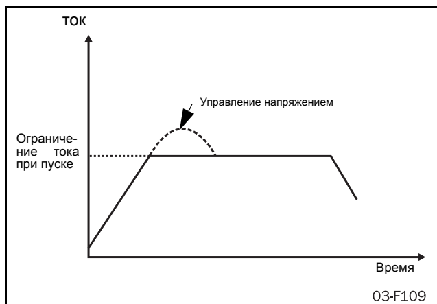
Рис. 34 Ограничение тока
