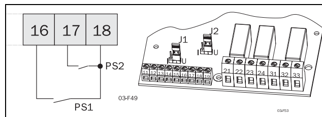
Рис. 56 Подключение сигналов управления
