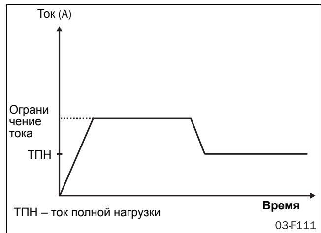
Рис. 4 Управление током
