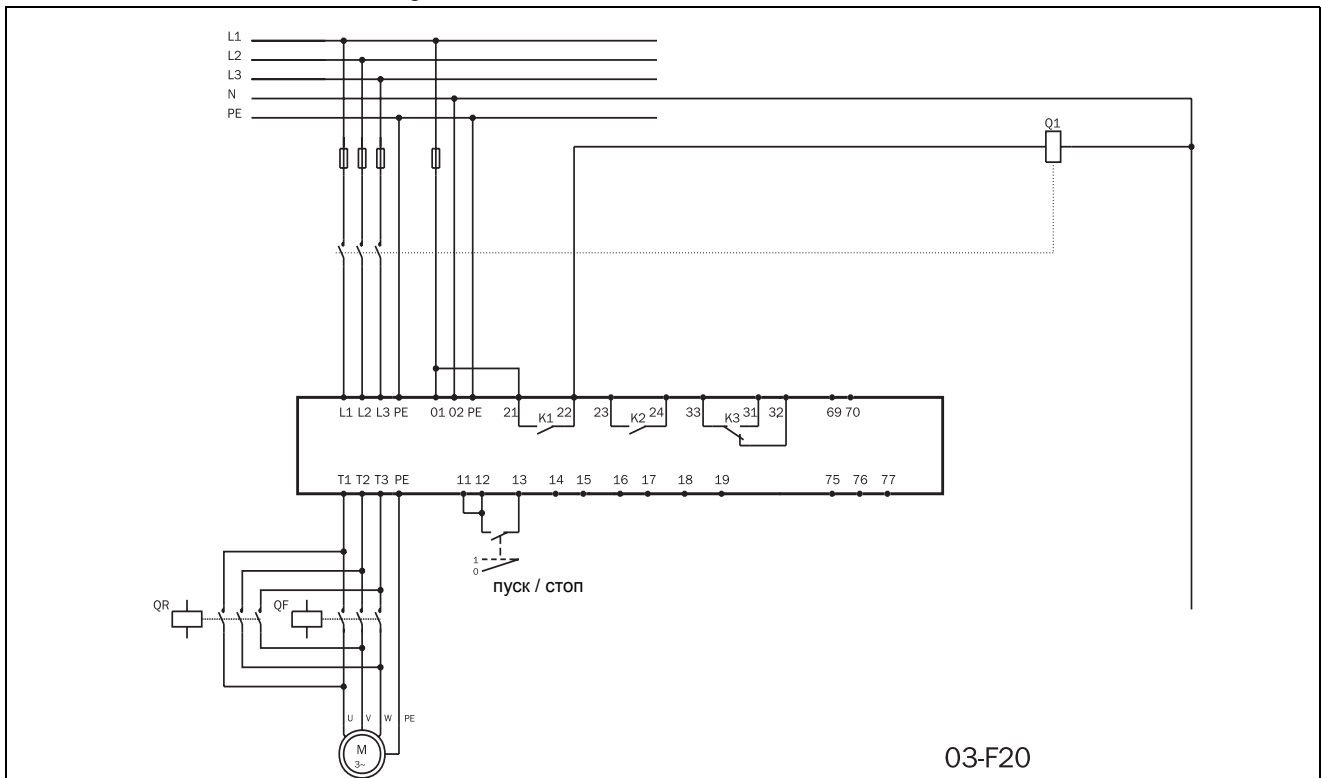
Рис. 31 Подключение с возможностью реверсирования.
