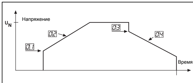
Рис. 32 Окна меню для времени пуска/останова, начального напряжения при пуске и сбросе напряжения при останове
