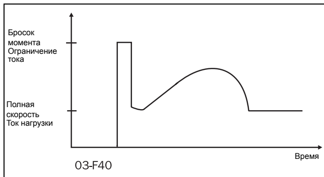
Рис. 42 Бросок момента при плавном пуске
