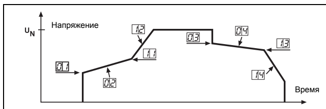
Рис. 33 Окна меню двойного наклона, начального напряжения при пуске и сбросе напряжения при останове
