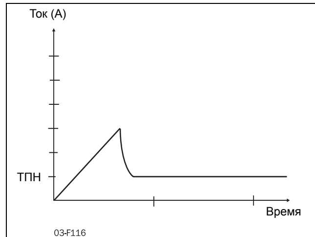
Рис. 3 Управление напряжением
