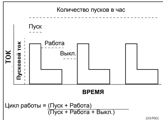
Рис. 9 Цикл работы, без шунтирования
