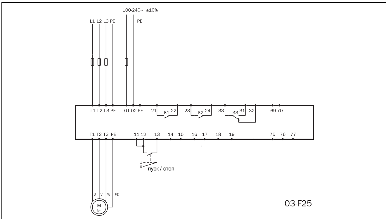
Рис. 29 Внешние цепи, стандартное подключение.
