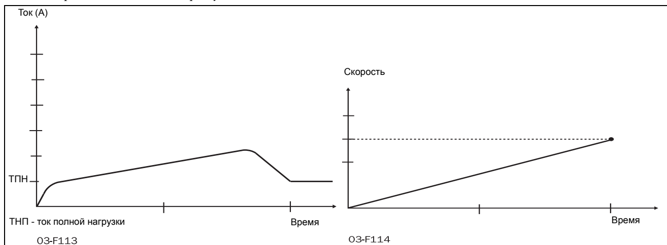
Рис. 41 Ток и скорость при управлении моментом
