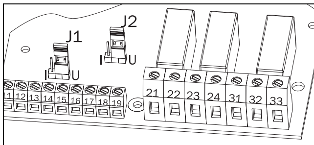
Рис. 53 Установка переключки J1 при выборе В / мА.
