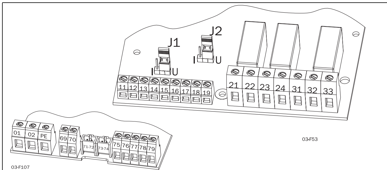
Рис. 28 Подключения на плате управления
