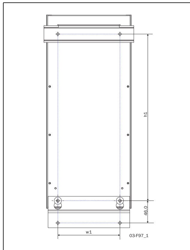
Рис. 17 Монтажные отверстия для MSF-017 ... MSF-250 (вид сзади).
