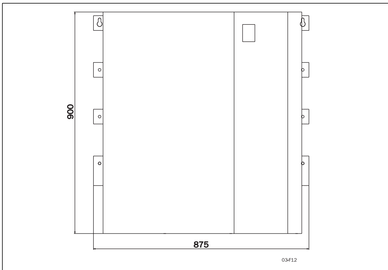
Рис. 22 MSF-1000 ... MSF-1400
