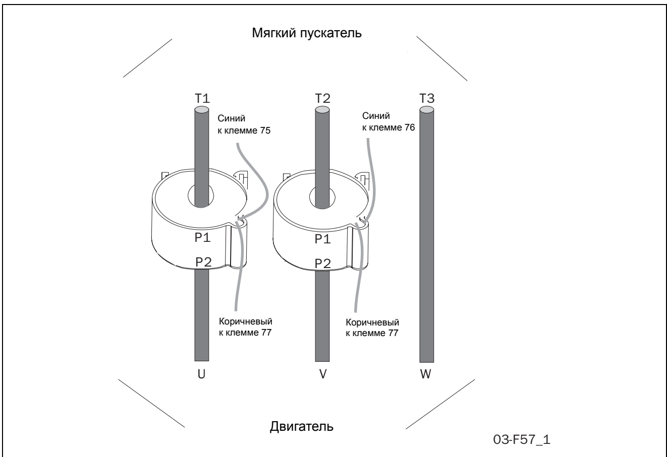
Рис. 45 Установка трансформаторов тока при шунтировании для MSF-310...MSF-1400.
