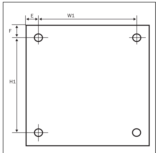
Рис. 20 Отверстия для винтов, MSF-310 ... MSF-835. Расстояния между отверстиями (мм)
