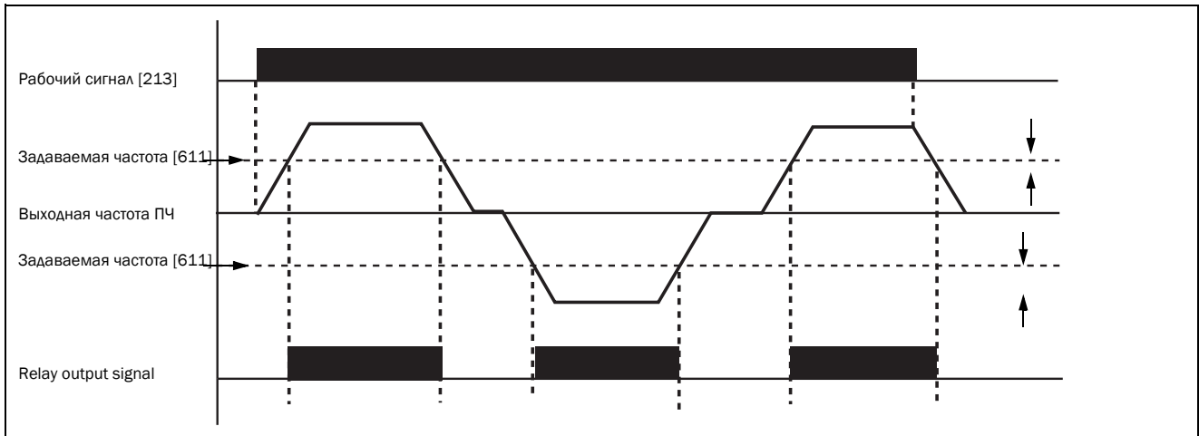
Рис. 37 Определение частоты [551]/[541]=3)
