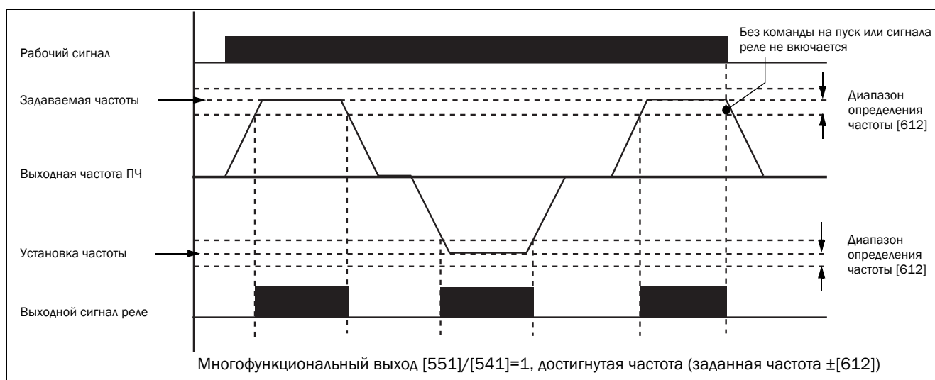
Рис. 35 Достижение заданной частоты, [551]/ [541]=1
