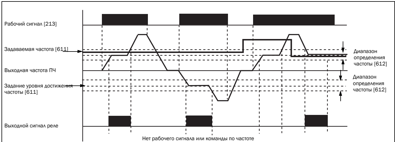
Рис. 36 Достижение частоты [551]/[541]=2
