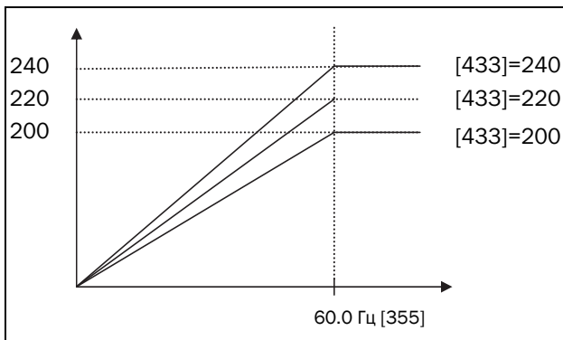
Рис. 32 В/Гц кривые при изменяющемся напряжении
