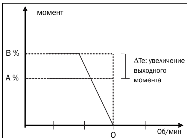
Рис. 27 Зависимость крутящий момент/скорость вращения
