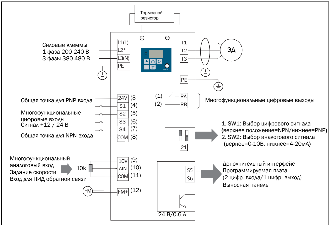
Рис. 10 Схема подключения
