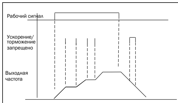
Рис. 33 Запрещение ускорения/торможения
