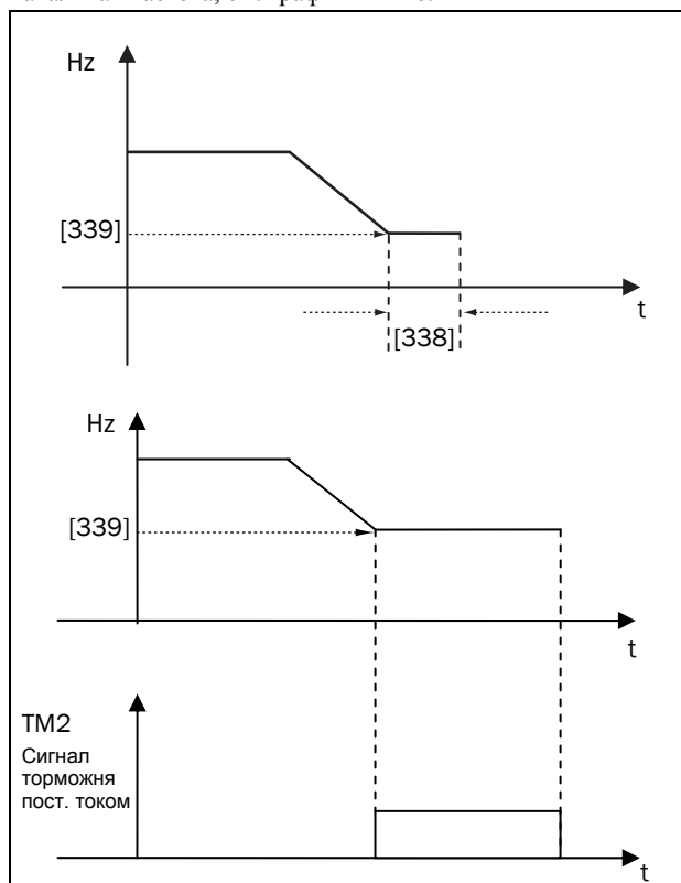
Рис. 24 Торможение постоянным током
