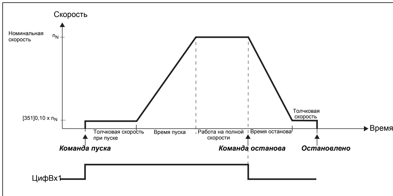
Рис. 48 Толчковая скорость при пуске и останове в течение выбранного периода времени.
