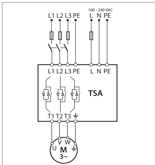
Рис. 11 Подключение сетевого питания двигателя и цепей управления
