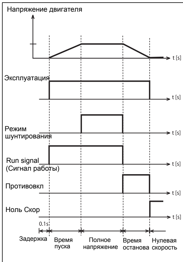
Рис. 63 Пример функции реле для цикла пуска и торможения.
