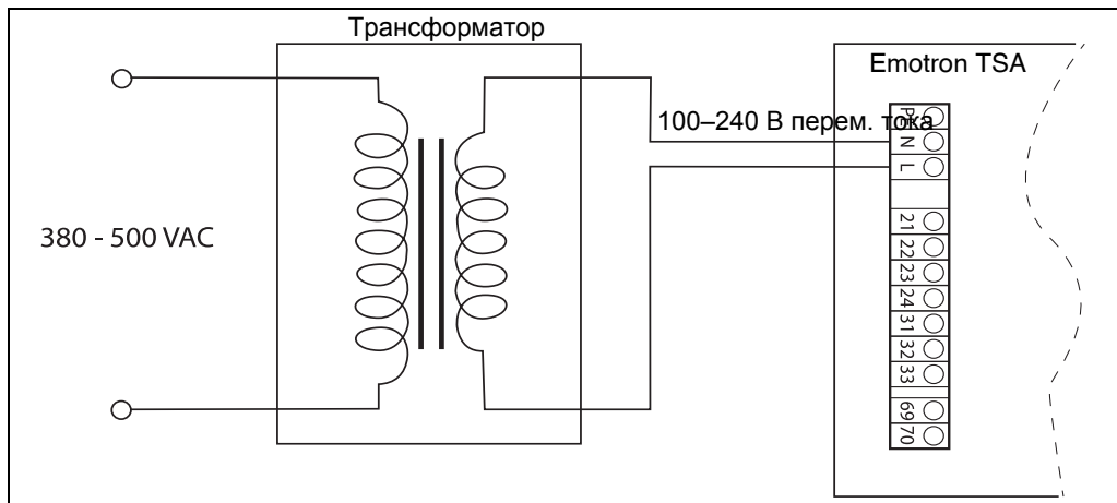
Рис. 27 Примерная схема при использовании трансформатора на 380–500 В переменного тока
