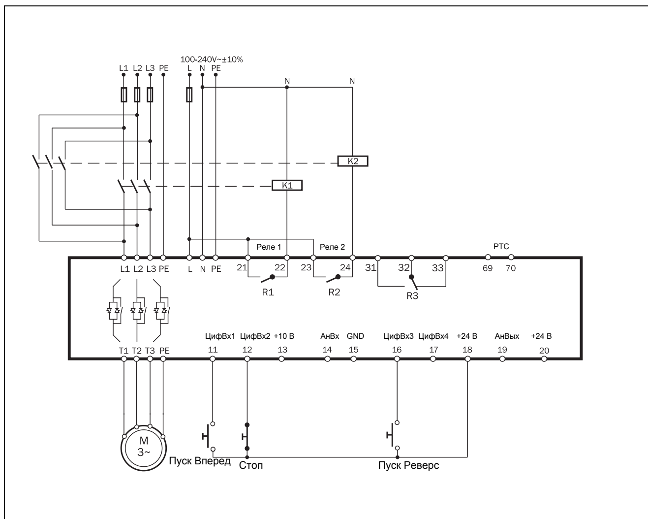
Рис. 25 Подключение для прямого/реверсного пуска.
