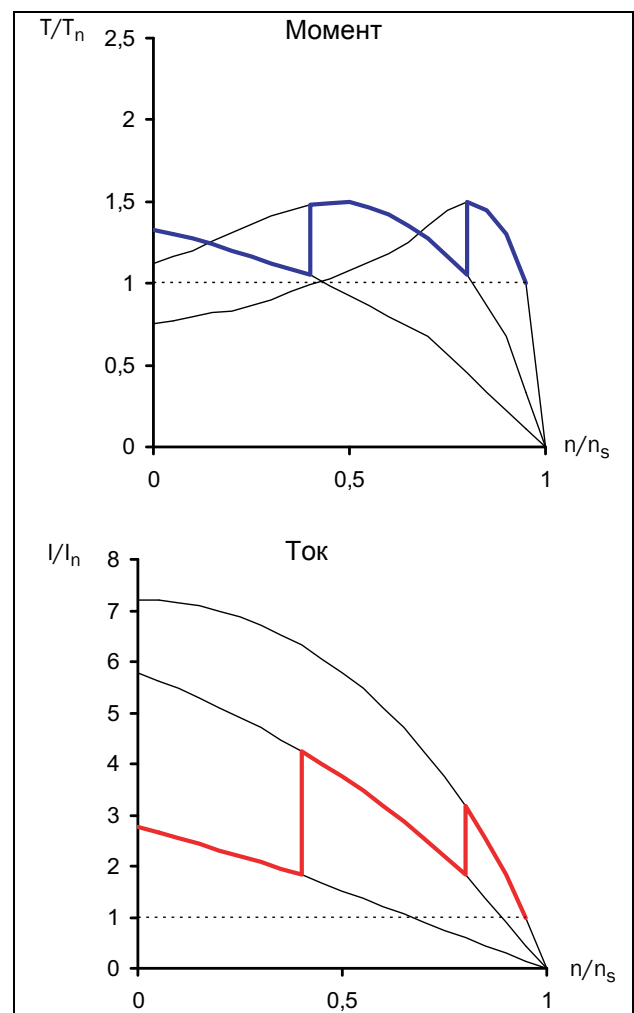
Рис. 91 Пуск с включением резистора в цепь ротора
