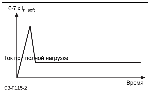
Рис. 53 Прямой пуск от сети (DOL).
