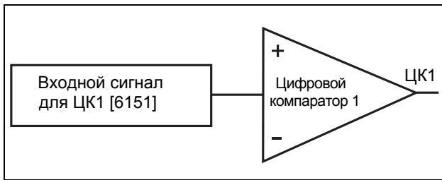
Рис. 69 Цифровой компаратор.
