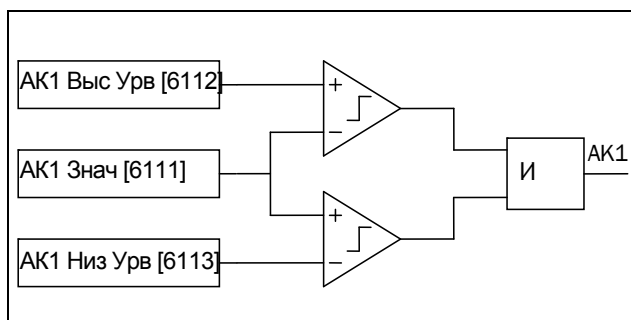
Рис. 65 Аналоговый компаратор двухпорогового типа
