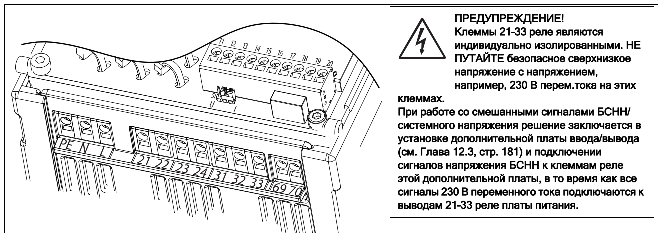
Рис. 18 Соединения платы управления и платы питания.
