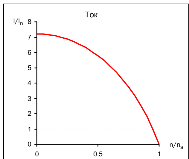
Рис. 84 Типичные характеристики тока при прямом пуске от сети
