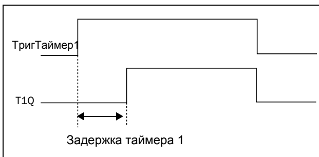
Рис. 70 Режим задержки таймера.
