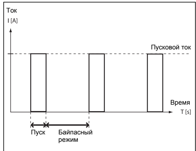
Рис. 26 Рабочий цикл.
