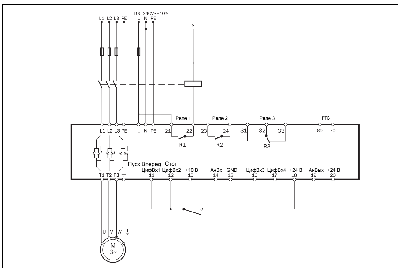
Рис. 21 Пример подключения проводки общих сигналов пуска-останова (2-проводное соединение).
