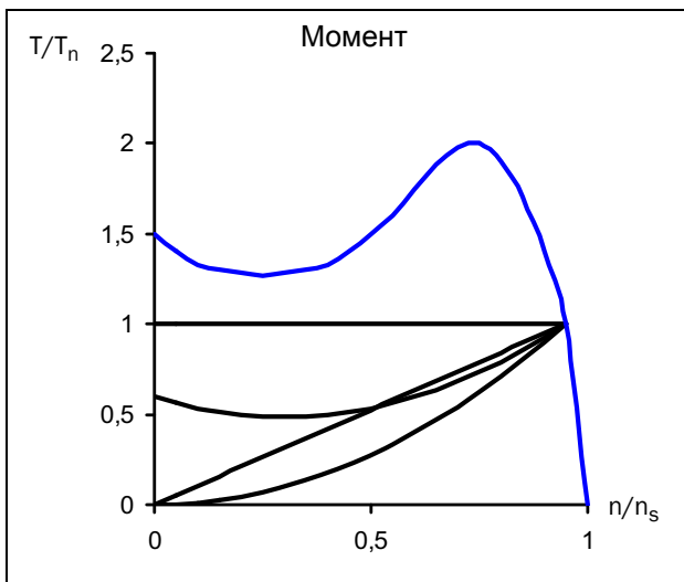
Рис. 85 Типичные характеристики момента нагрузки
