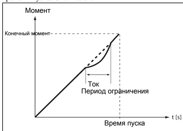
Рис. 54 Увеличение момента в период ограничения тока.
