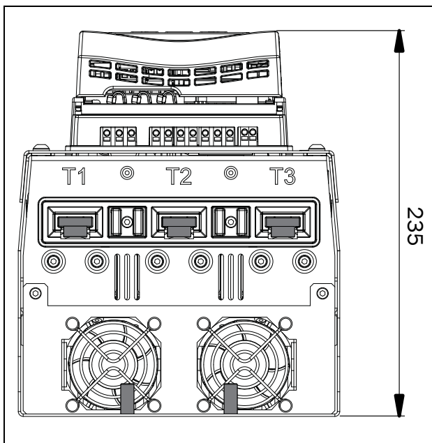
Рис. 5 Габаритные размеры Emotron TSA типоразмера 3, вид снизу.
