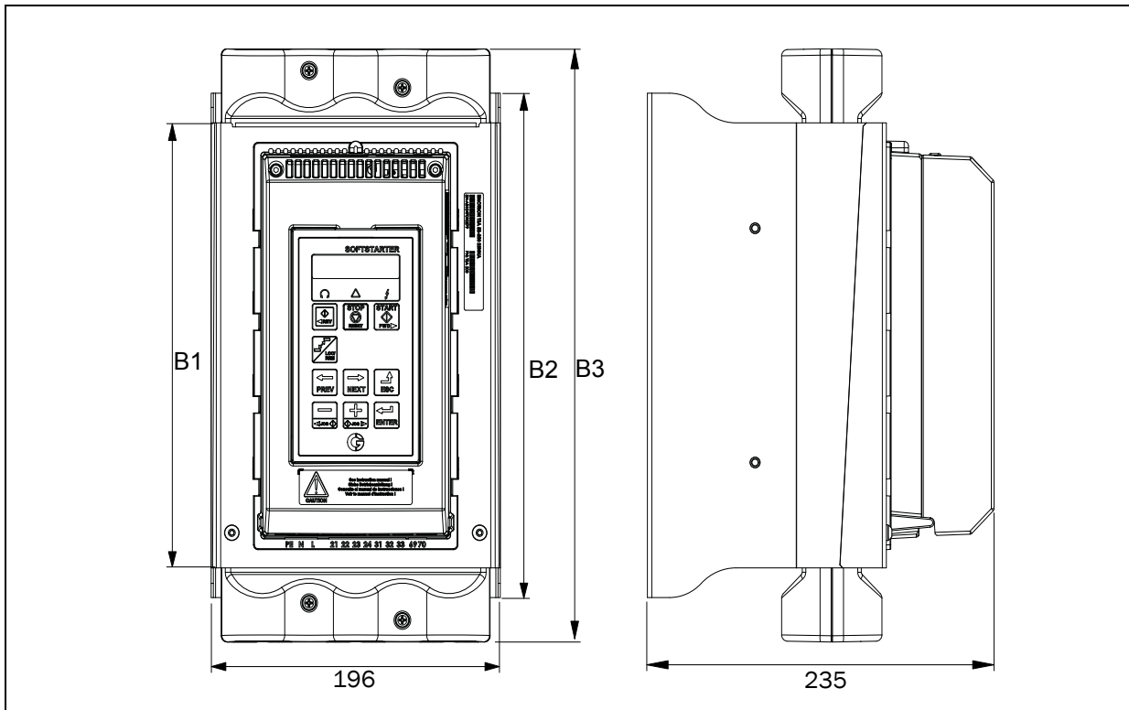
Рис. 4 Габаритные размеры Emotron TSA типоразмера 3.
