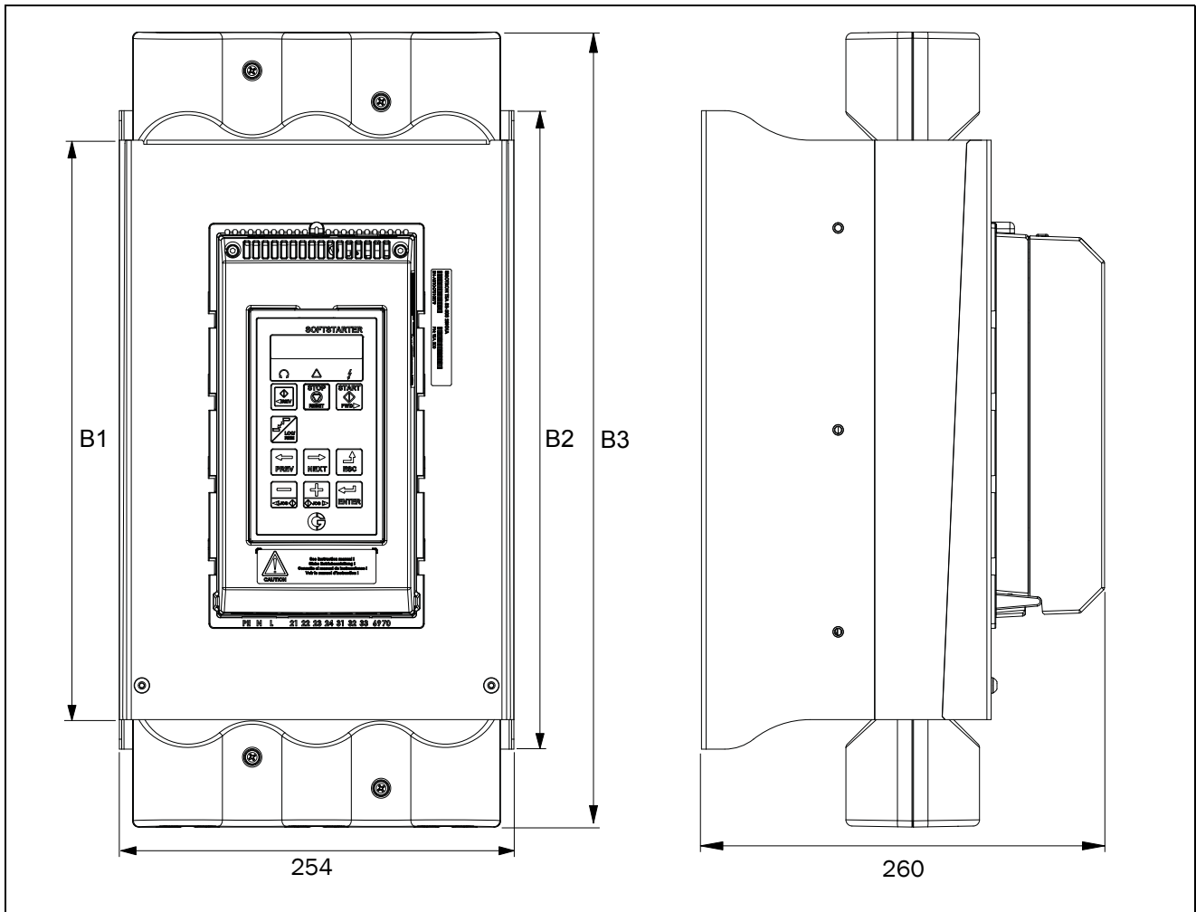
Рис. 6 Габаритные размеры Emotron TSA типоразмера 4.
