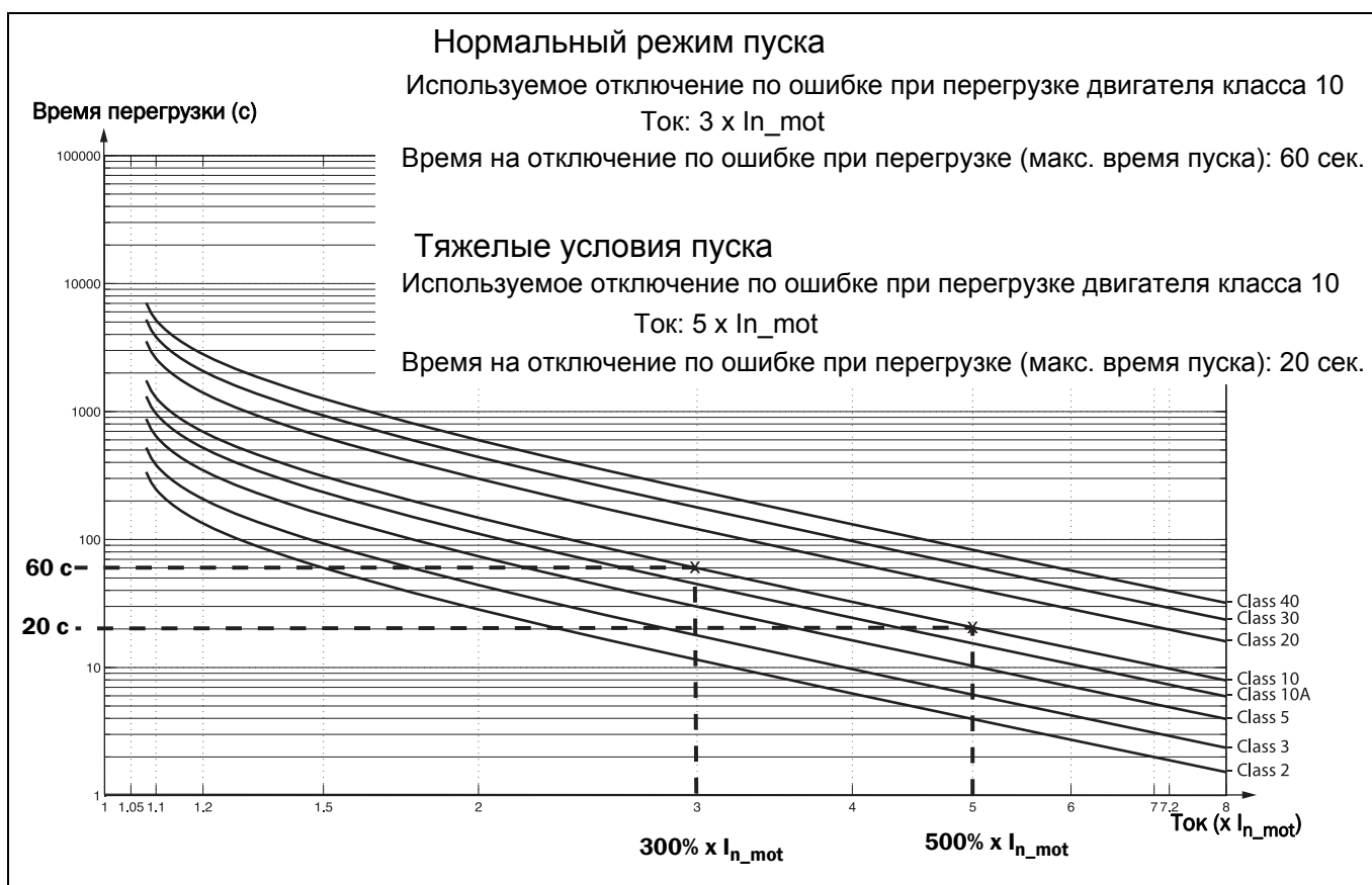
Рис. 50 Кривая нагрева
