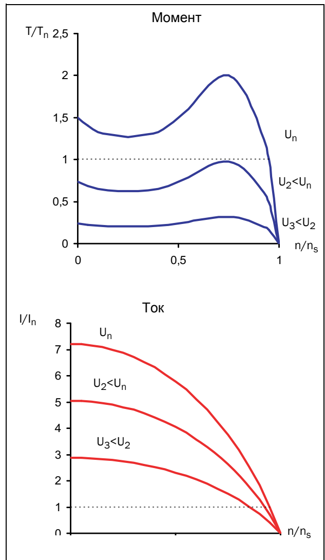
Рис. 86 Пониженное напряжение при пуске
