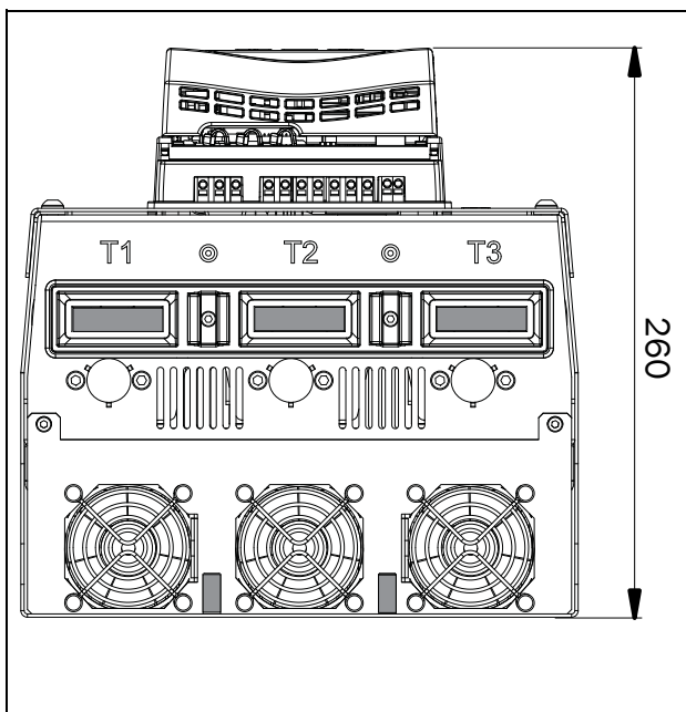
Рис. 7 Габаритные размеры Emotron TSA типоразмера 4, вид снизу.
