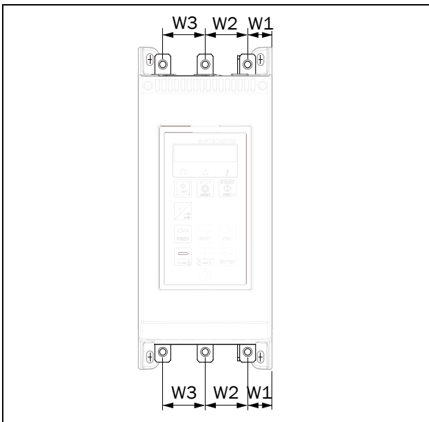
Рис. 15 Чертеж общего вида расстояний между шинами
