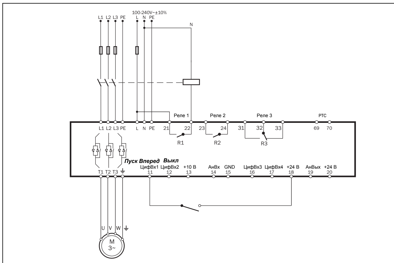
Рис. 22 Пример подключения общих сигналов пуска-останова (2-проводное соединение), управление по уровню.
