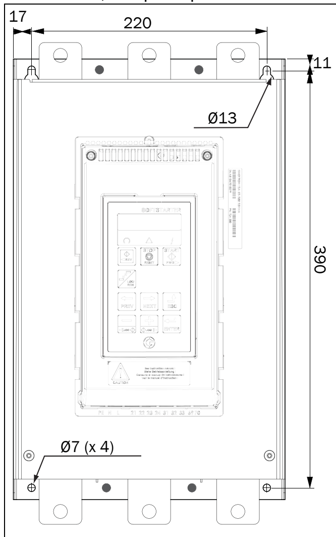
Рис. 10 Расположение отверстий Emotron TSA, типоразмер 4.
