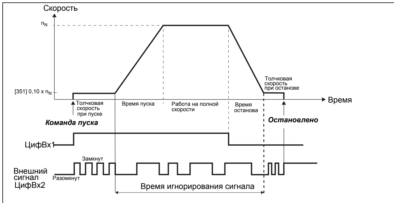
Рис. 47 Толчковая скорость, управляемая по внешнему импульсному сигналу.
