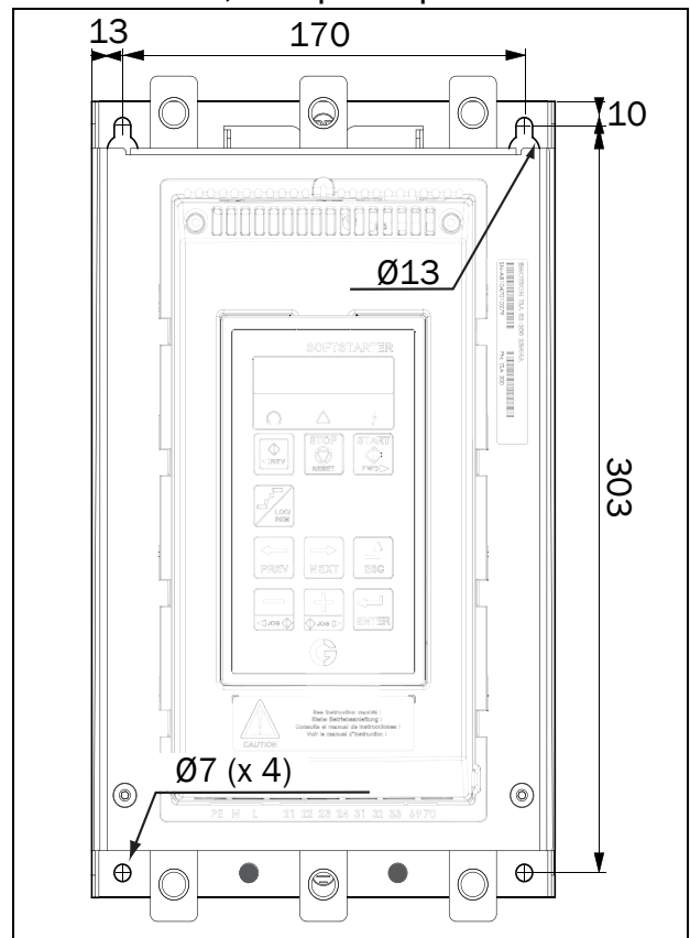
Рис. 9 Расположение отверстий Emotron TSA, типоразмер 3.
