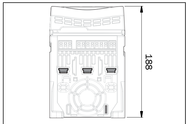
Рис. 3 Габаритные размеры Emotron TSA типоразмеров 1 и 2, вид снизу.
