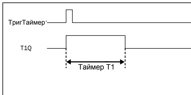
Рис. 72 Режим включения таймера.
