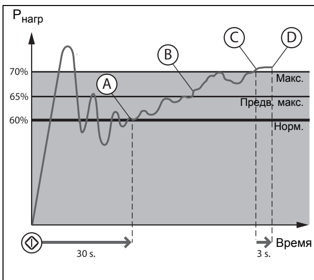
Рис. 43 Пример 2. Автонастройка функции монитора нагрузки.
