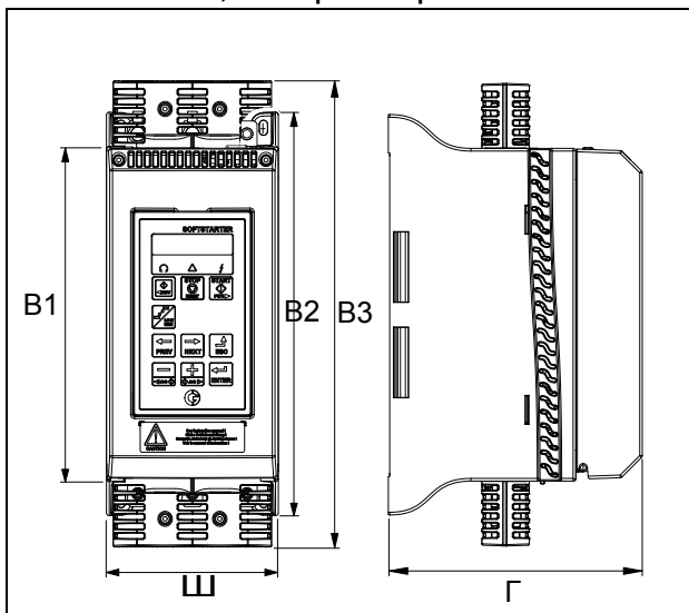
Рис. 2 Габаритные размеры Emotron TSA типоразмеров 1 и 2.
