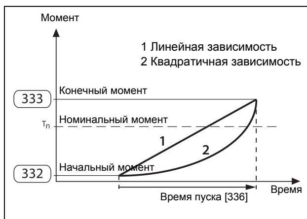
Рис. 51 Управление моментом при пуске
