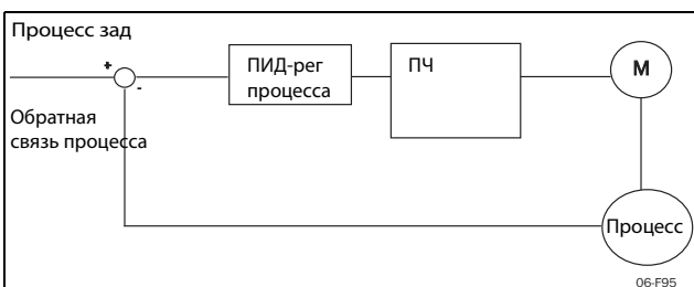
Рис. 103 Замкнутый контур ПИД-регулирования
