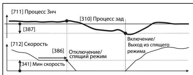
Рис. 104 Отключение/спящий режим ПИД при обычном ПИД-регулировании
