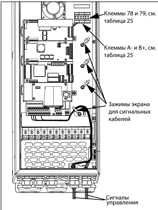
Рис. 61 Подключение кабелей управления, модели VFX от 061 до 074, типоразмер D, и модели от 69-033 до 69-058, типоразмер D(69)
