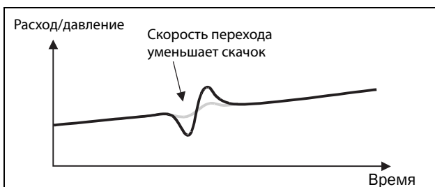
Рис. 112 Эффект использования скорости перехода
