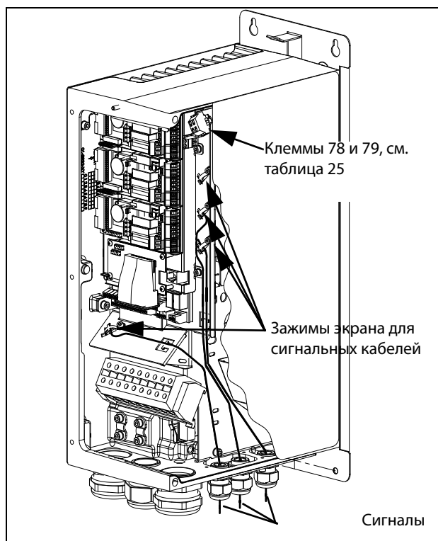
Рис. 59 Подключение кабелей управления, модели VFX от 026 до 046, типоразмер В
