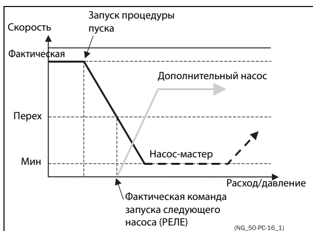
Рис. 111 Скорость перехода
