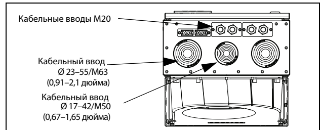
Рис. 21 Кабельный интерфейс для подключения электрической сети, электродвигателя, DC+/DC-, тормозного резистора и связи, устройство Emotron VFX модели с 48-210 по 295 (типоразмер F), устройство Emotron VFX модели с 69-082 по 200 (типоразмер F69)
