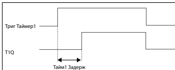
Рис. 131 Режим задержки таймера.
