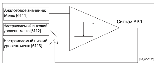
Рис. 124 Аналоговый компаратор гистерезисного типа
