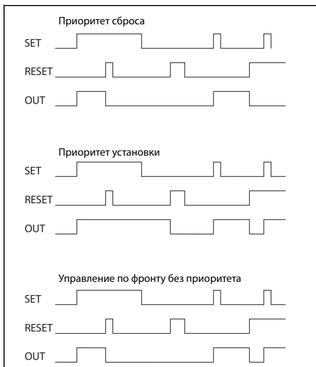
Рис. 134 Программируемые режимы триггера.
