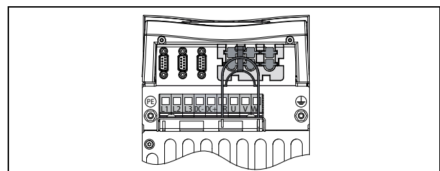
Рис. 11 Вид снизу, устройство Emotron VFX модели 48-025 до 48-058 (типоразмер С2), модели 69-002 до 69-025 (типоразмер С2(69)), с кабельным интерфейсом для подключения электрической сети, электродвигателя, опции DC+/DC-, тормозного резистора и управления
