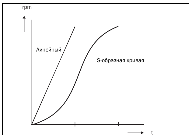
Рис. 93 Форма кривой разгона
