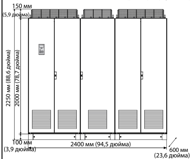
Устройство Emotron VFX48: модель 2K0 (размер корпуса M) Устройство Emotron VFX69: модель 1K6 (размер корпуса M69)
