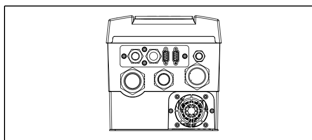
Рис. 7 Пример устройства Emotron VFX модели 48/52-003 — 018 (размер корпуса В) с дополнительными интерфейсом CRIO и разъемами D-sub
