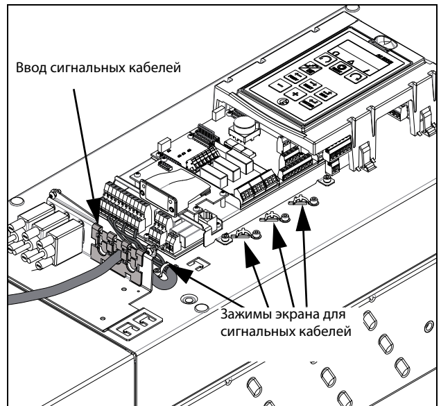
Рис. 64 Подключение кабелей управления, модели VFX от 48-142 до 48-365, типоразмеры E2, F2 и FA2 (принципиальная схема)
