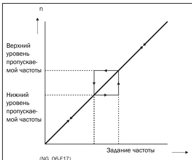
Рис. 98 Пропускаемая частота.
