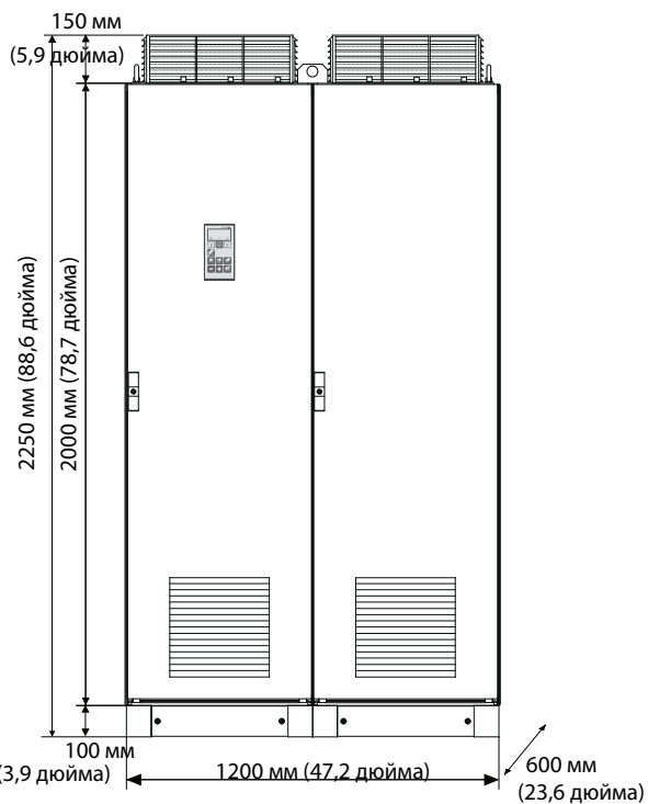
Устройство Emotron VFX48: модели 860 до 1K0 (типоразмер J) Устройство Emotron VFX69: модели 650–800 (размер корпуса J69)
