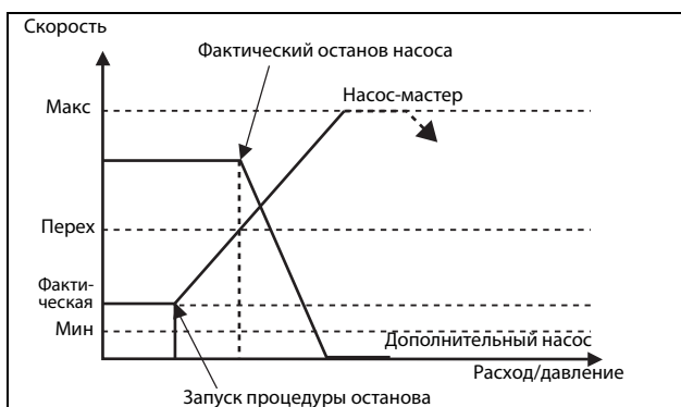
Рис. 113 Скорость перехода при останове
