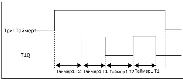
Рис. 132 Альтернативный режим таймера
