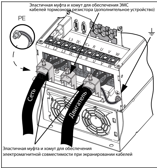
Рис. 36 Подключение сетевого питания и двигателя, модели от 48-060 до 48-105, размер корпуса D2 и модели 69-033 — 69-058, размер корпуса D2(69)
