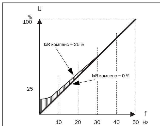
Рис. 100 IxR Компенс при линейной зависимости В/Гц
