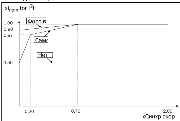
Рис. 86 Кривые I^2t
