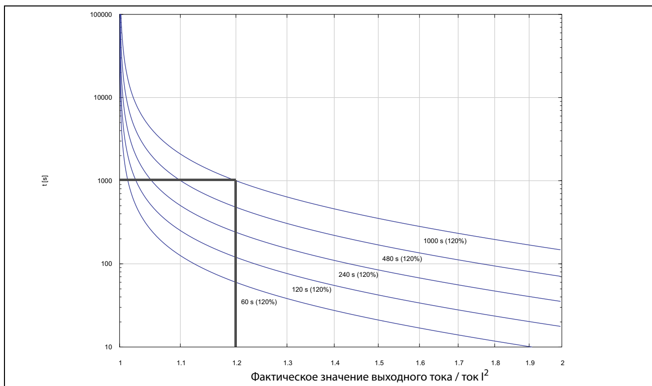
Рис. 87 Функция I^2t
