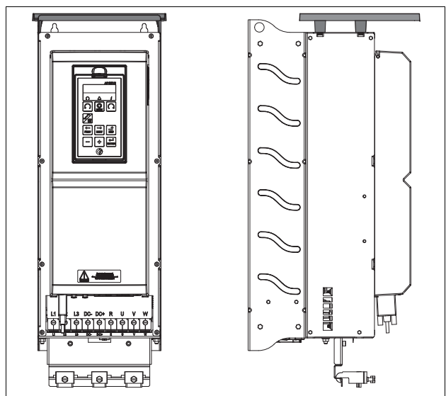
Рис. 154 Дополнительная верхняя крышка, установленная на корпусе размера D2
