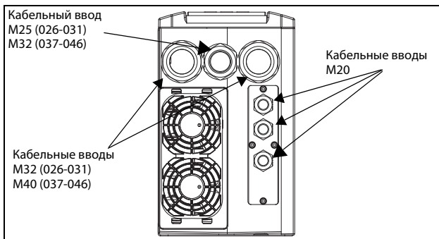
Рис. 9 Кабельный интерфейс для подключения электрической сети, электродвигателя и интерфейсов связи, Emotron VFX моделей 48/52-026 до 046 (типоразмер В)
