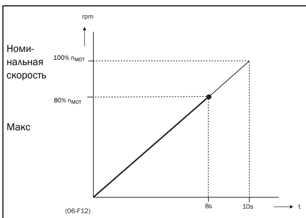
Рис. 90 Время разгона и максимальная скорость
