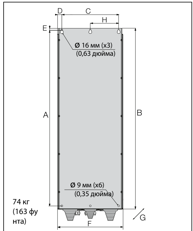
Рис. 20 Emotron VFX модели 48-210 до 295 (типоразмер F), Emotron VFX модели 69-82 до 200 (типоразмер F69)
