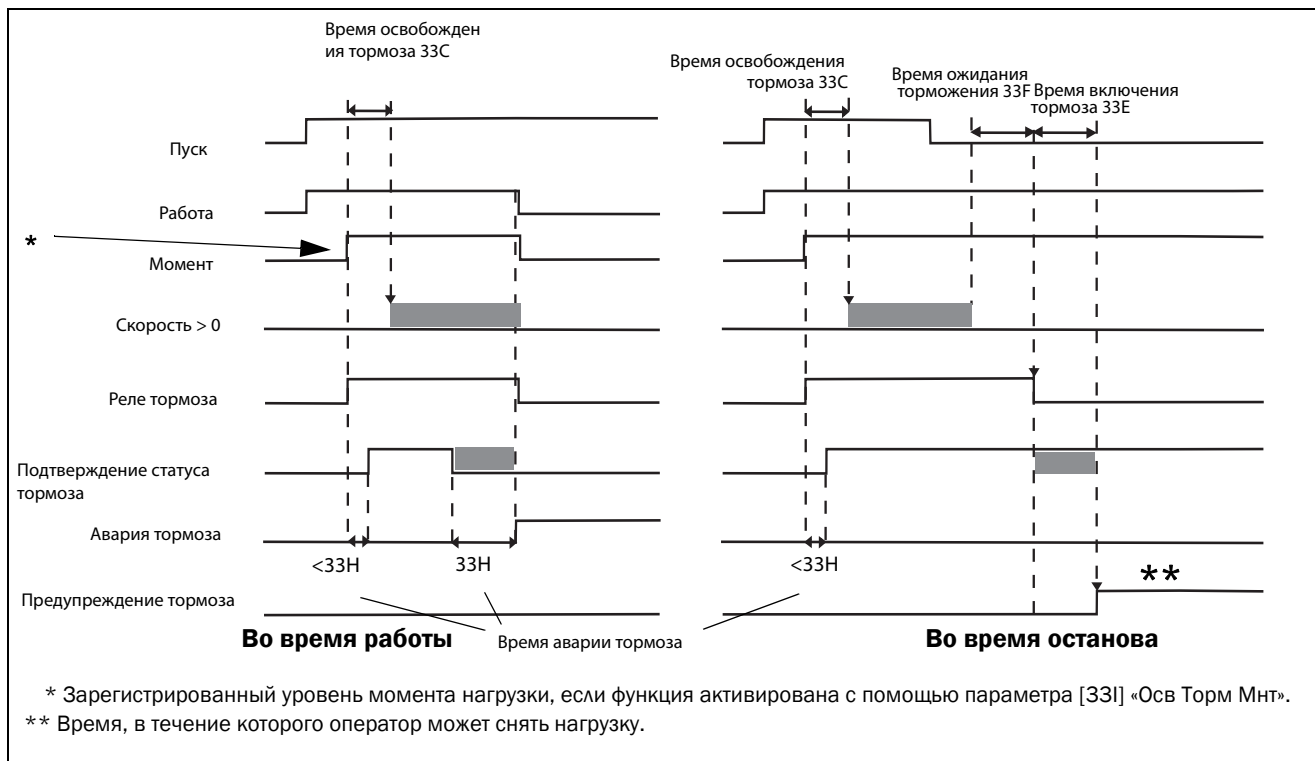
Рис. 96 Принцип работы тормоза при аварии в процессе работы и во время останова
