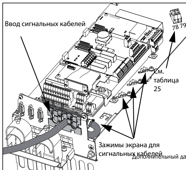
Рис. 60 Подключение кабелей управления, модели VFX от 48-025 до 48-058, типоразмер С2, и модели от 69-002 до 69-025, типоразмер С2(69)
