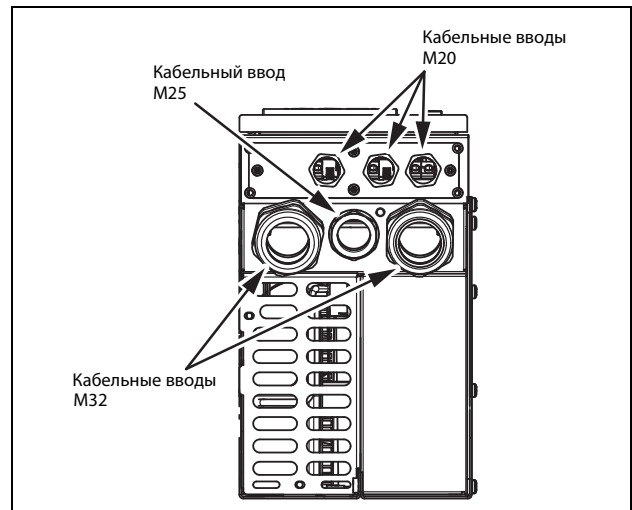
Рис. 13 Кабельный интерфейс для подключения электрической сети, электродвигателя и интерфейсов связи, Emotron VFX модели 69-002 до 025 (типоразмер С69)
