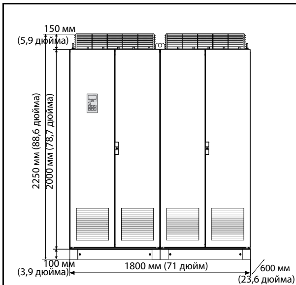
Устройство Emotron VFX48: модели от 1K35 до 1K5 (размер корпуса K) Устройство Emotron VFX69: модель 1K2 (размер корпуса K69)
