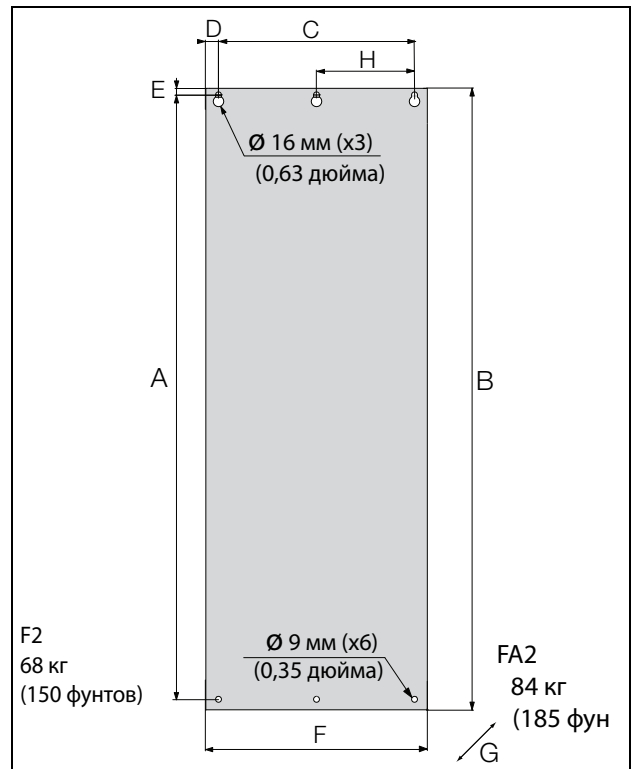
Рис. 24 Emotron VFX/ модели 48-205 до 48-293 (типоразмер F2) и 48-365-20 (типоразмер FA2)
