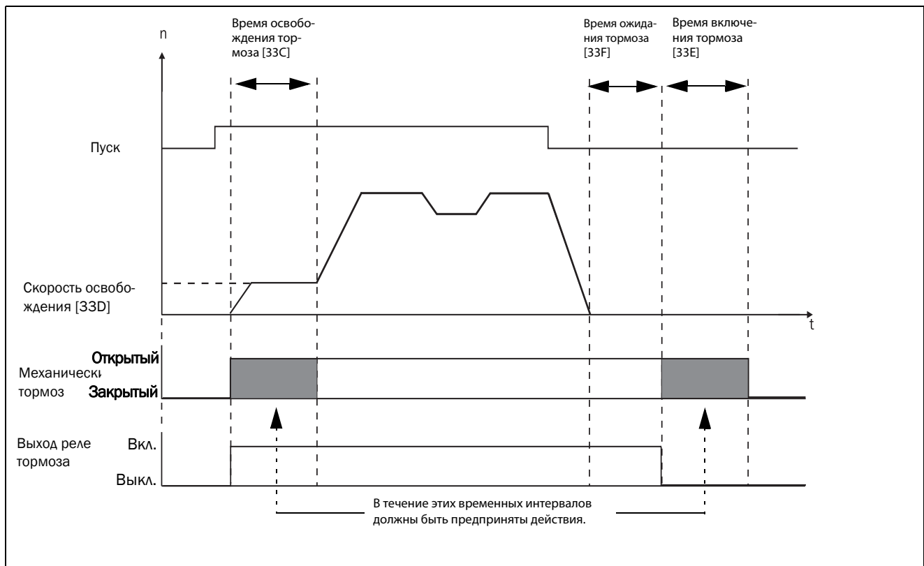
Рис. 95 Функции торможения.
