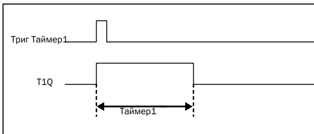
Рис. 133 Режим включения таймера.
