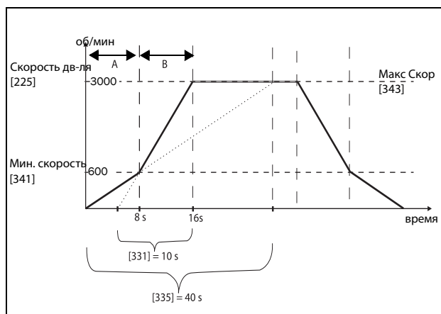
Рис. 92 Пример расчета времени разгона (графические данные не пропорциональны).
