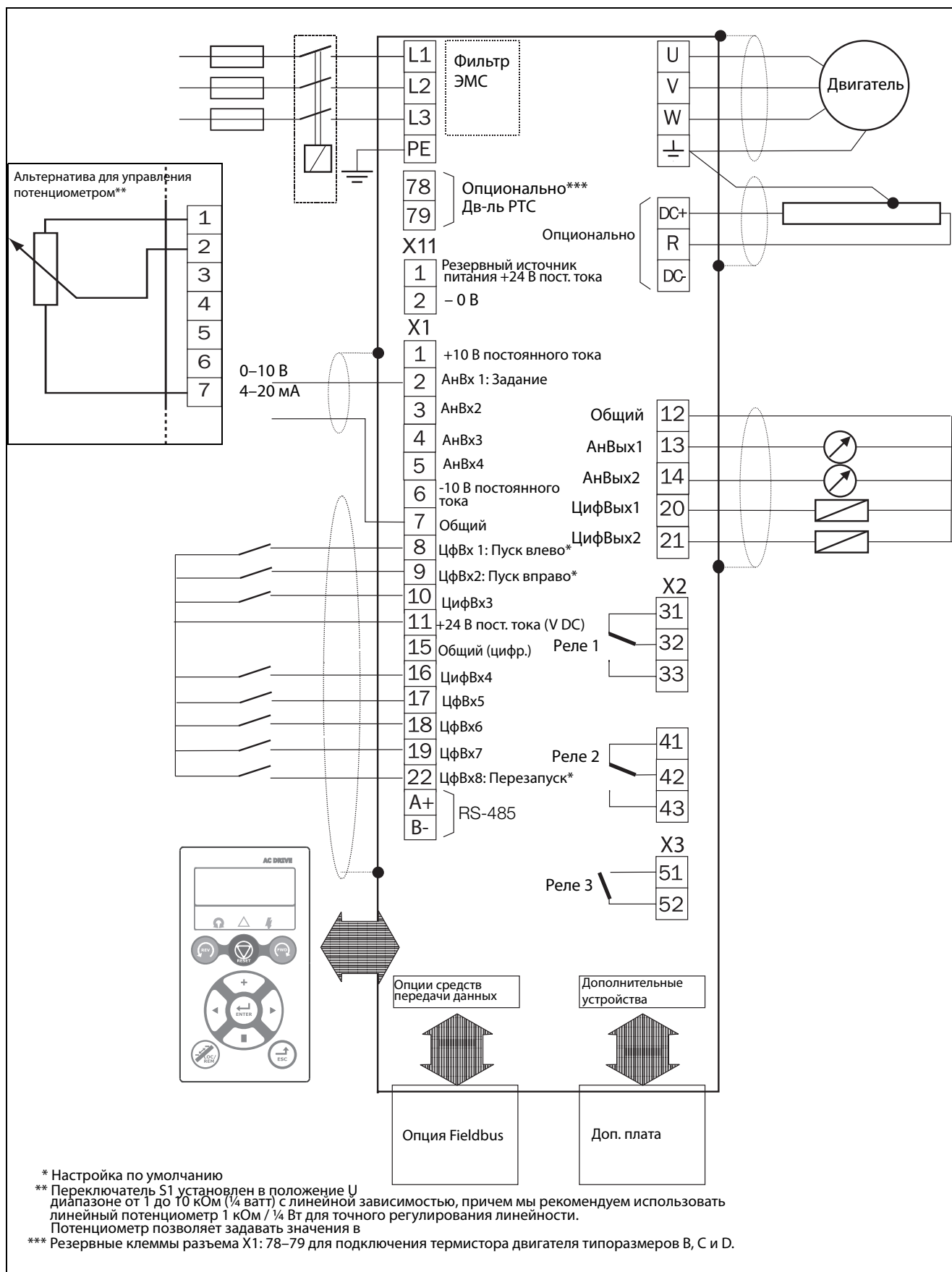
Рис. 57 Пример подключения
