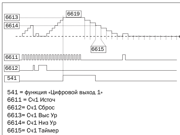
Рис. 135 Счетчики, принцип действия.
