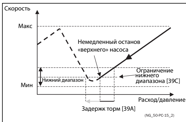
Рис. 110 Ограничение нижнего диапазона
