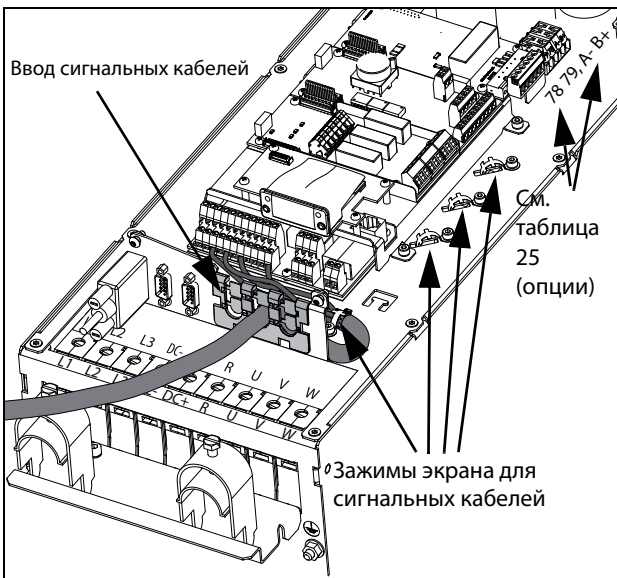
Рис. 62 Подключение кабелей управления, модели от VFX 48-060 до 48-105, типоразмер D2, и модели от 69-033 до 69-058, типоразмер D2(69)
