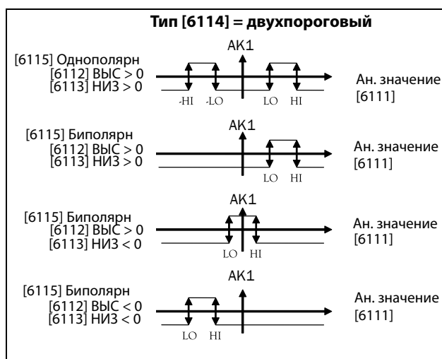
Рис. 129 Основные функции компаратора для «Тип [6114] = двухпороговый» и «Полярный [6115]».
