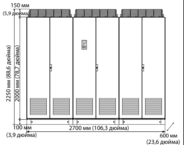
Устройство Emotron VFX48: модель 2K25 (размер корпуса N) Устройство Emotron VFX69: модель 1K8 (размер корпуса N69)
