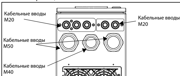
Рис. 15 Кабельный интерфейс для подключения электрической сети, электродвигателя и интерфейсов связи, Emotron VFX модели 48/52-061 до 074 (типоразмер D), модели 69-033 до 69-058 (типоразмер D69)
