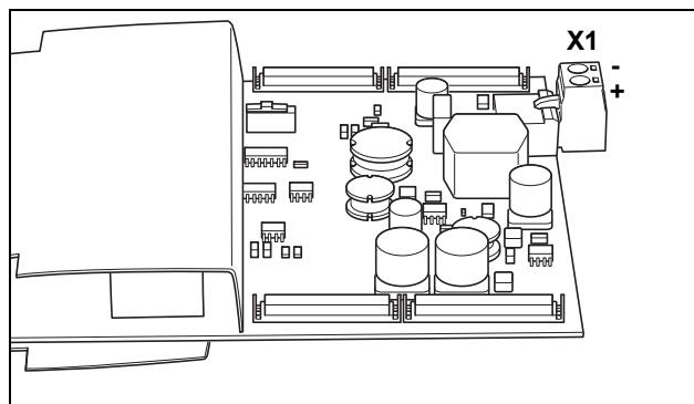
Рис. 153 Плата резервного источника питания с цепью измерения напряжения постоянного тока с гальванической развязкой, для ПЧ морского исполнения типоразмеров В-D и F69-T69
