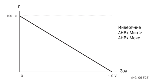
Рис. 121 Инвертирование сигнала задания
