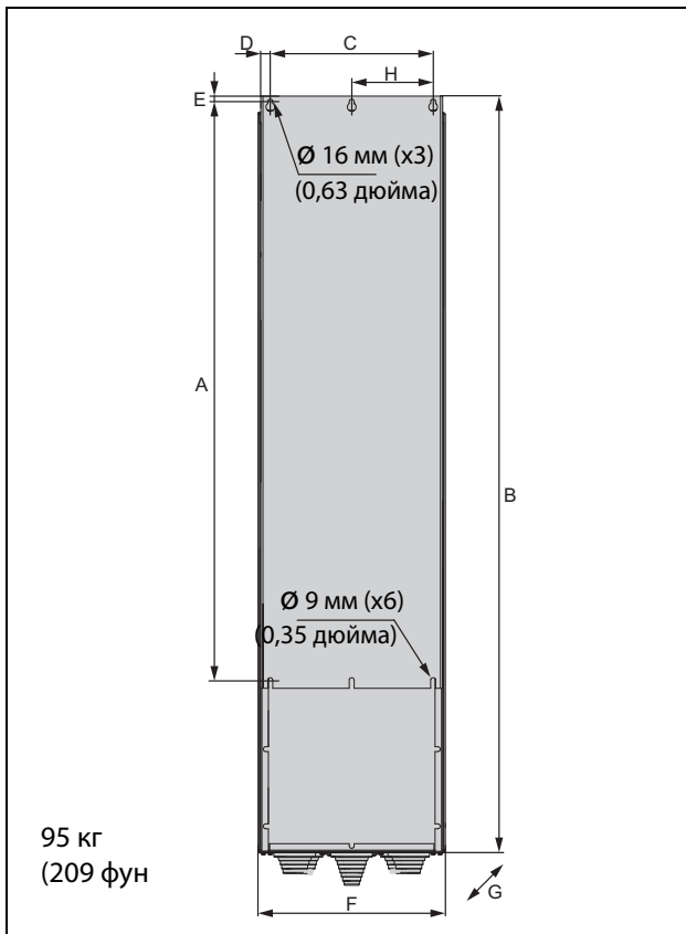
Рис. 25 Emotron VFX модель 48-365-54 (типоразмер FA)
