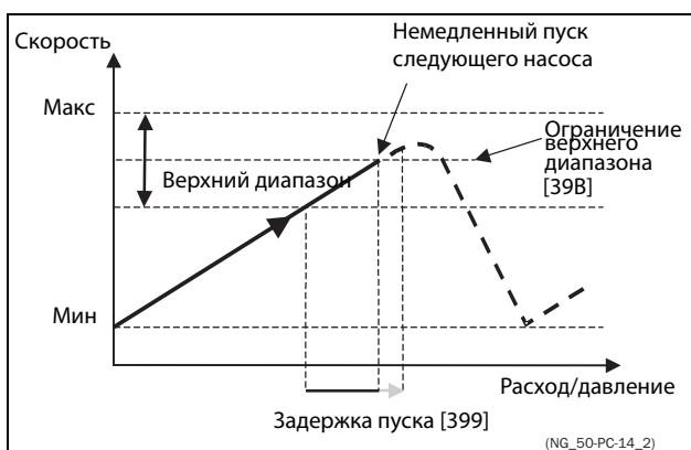
Рис. 109 Ограничение верхнего диапазона
