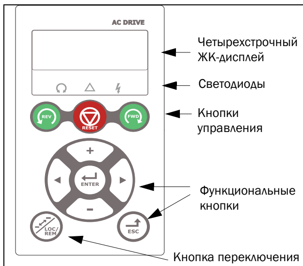
Рис. 78 Панель управления с четырехстрочным дисплеем, светодиодными индикаторами и кнопками
