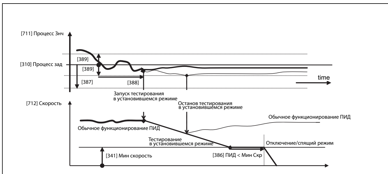
Рис. 106 Тестирование в установившемся режиме
