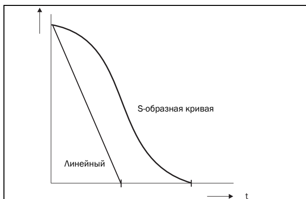
Рис. 94 Форма кривой торможения
