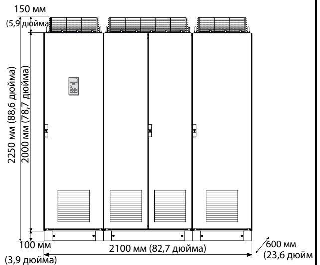
Устройство Emotron VFX48: модель 1K75 (размер корпуса L) Устройство Emotron VFX69: модель 1K4 (размер корпуса L69)
