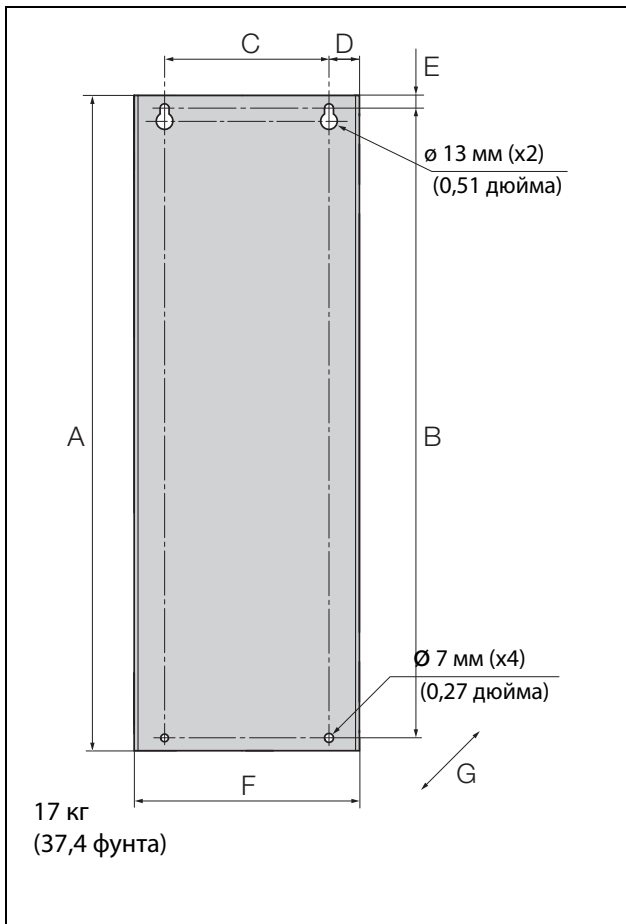
Рис. 12 Emotron VFX модели 69-002 до 025 (типоразмер С69)
