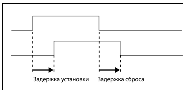
Рис. 130 Задержка установки/сброса выходного сигнала
