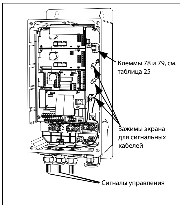
Рис. 58 Подключение кабелей управления, модели VFX от 003 до 018, типоразмер В
