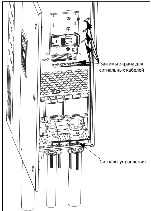
Рис. 63 Подключение кабелей управления, модели VFX от 48-090 до 295 и модели VFX от 69-82 до 200, типоразмер E, F и F69 (принципиальная схема)
